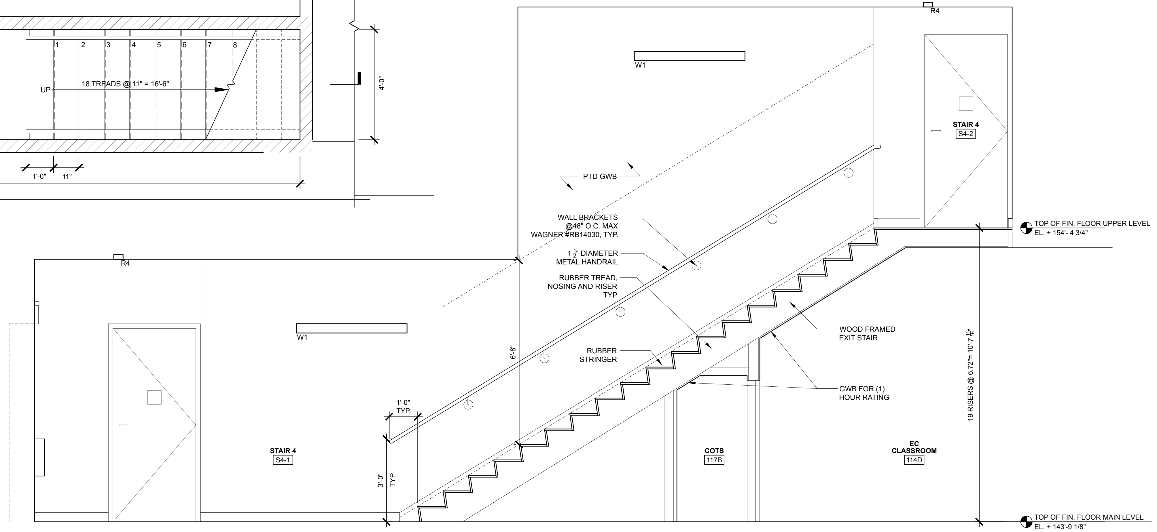
3 STAIR S4 SECTION SCALE: 1/2" = 1'-0"
