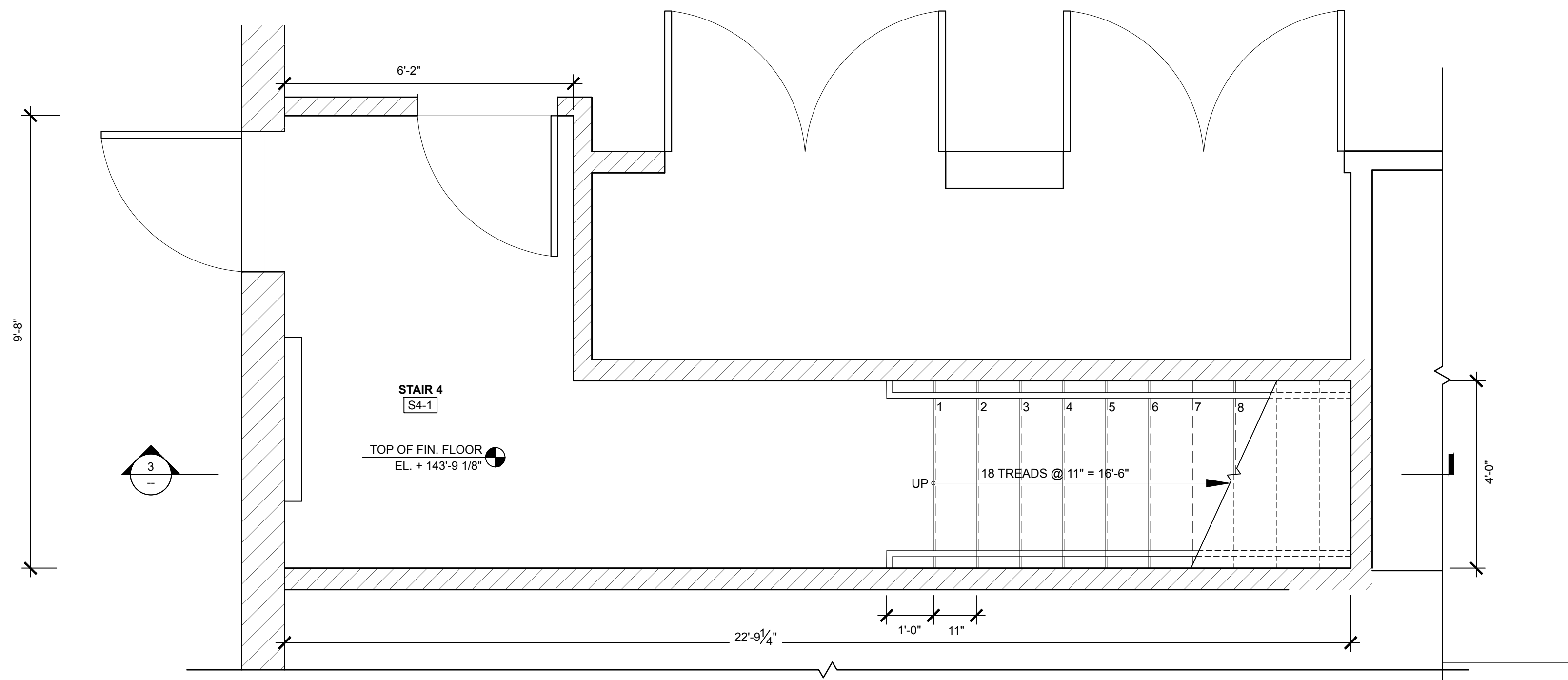
2 STAIR S4-1 UPPER LEVEL SCALE: 1/2" = 1'-0"
