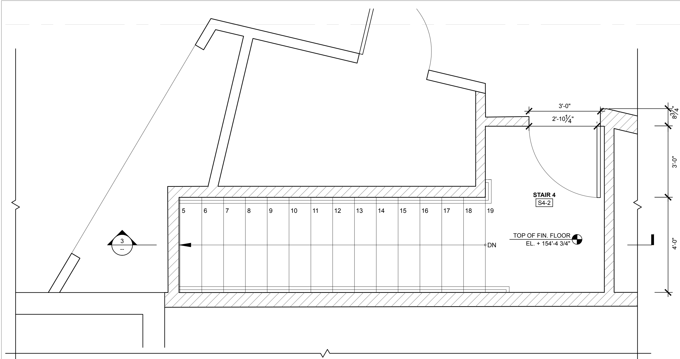
1 STAIR S4-2 UPPER LEVEL SCALE: 1/2" = 1'-0"
