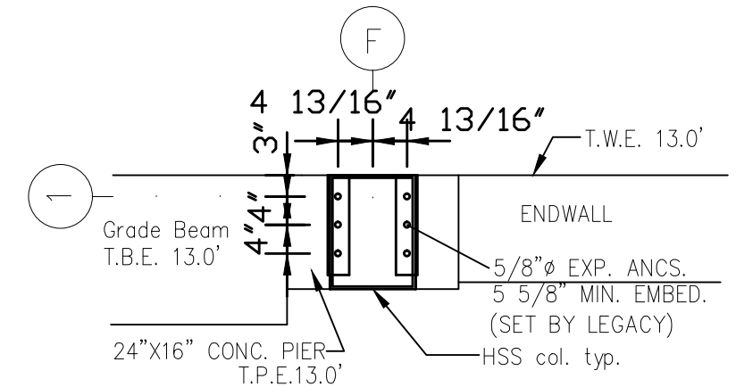
E Baseplate E 1/2"=1'-0"
