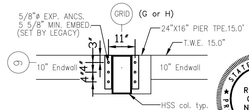
I Baseplate I 1/2"=1'-0"
