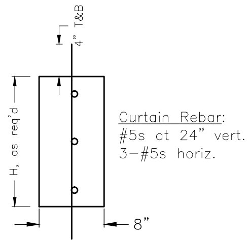
CURTAIN WALL (typ UNO)
