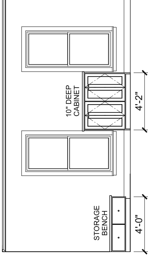
Elevation 4
