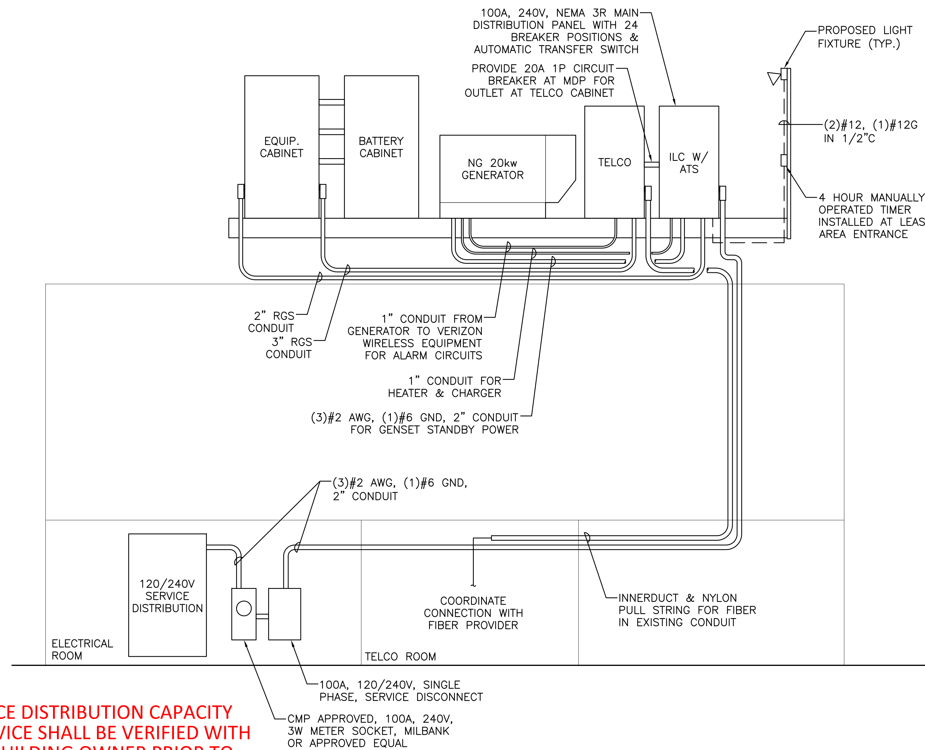
1 POWER RISER DIAGRAM SCALE: N.T.S.
