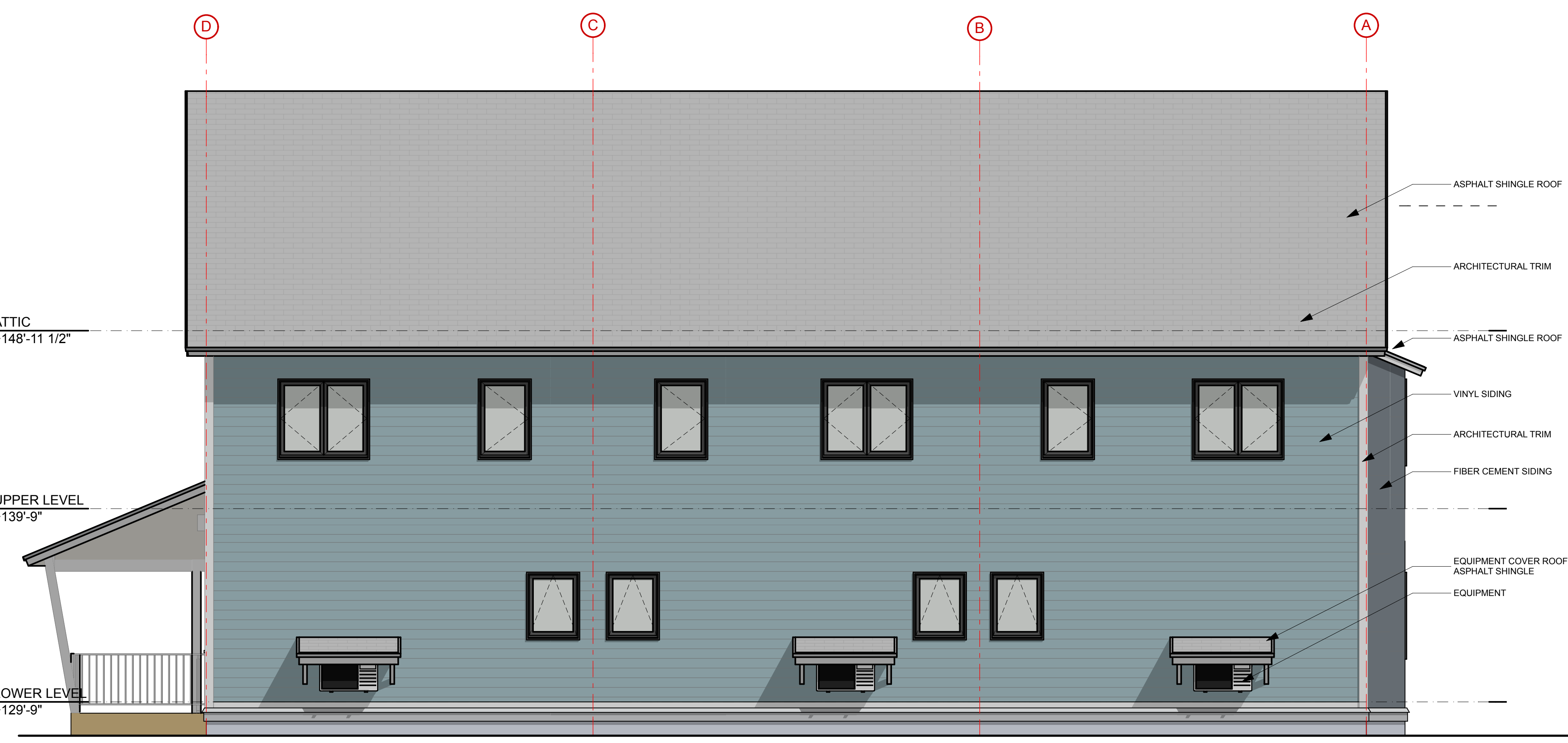
1 NW ELEVATION SCALE: 1/4" = 1'-0"
