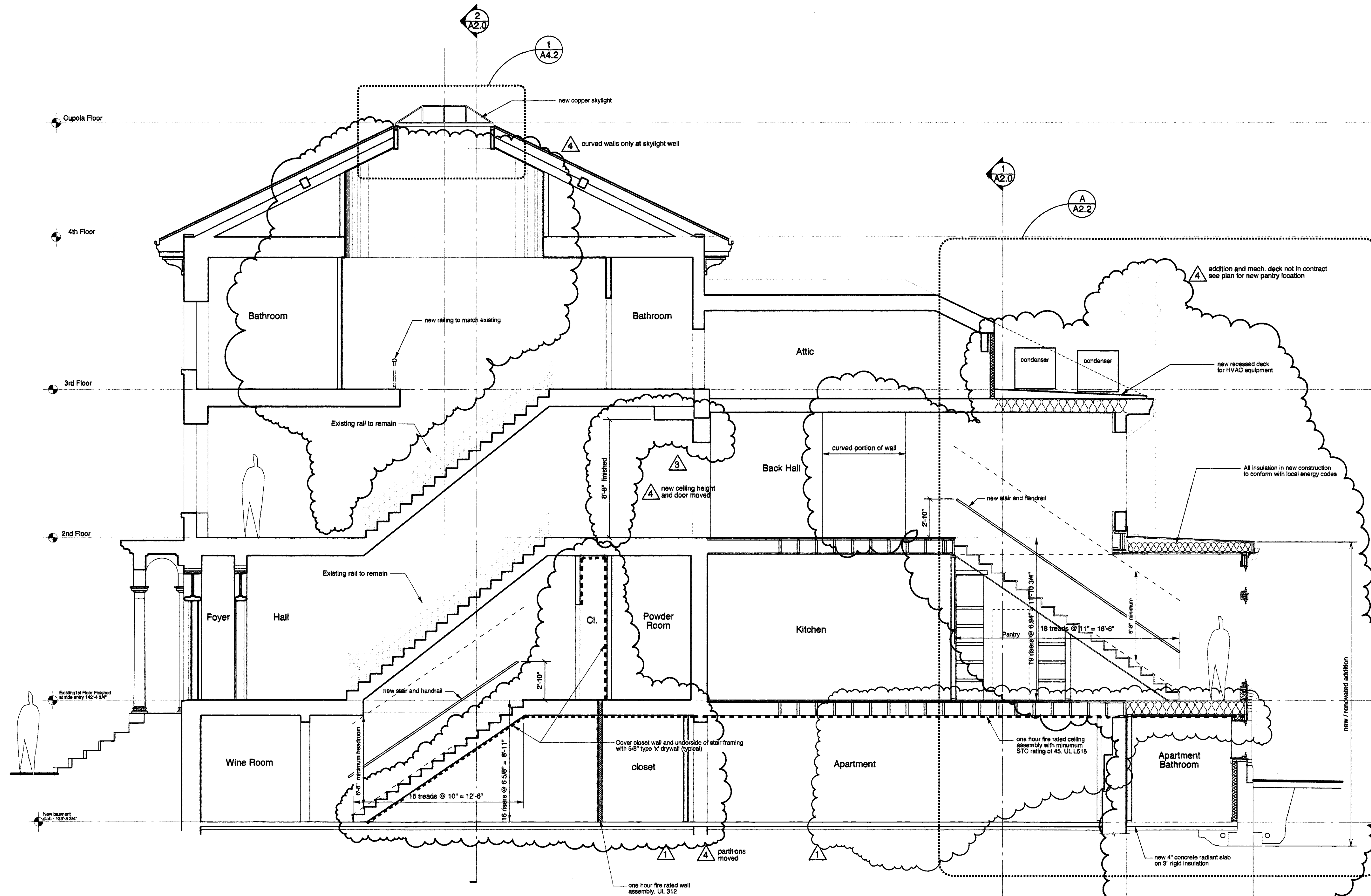
Section 3 SCALE: 1/4" = 1'-0"
