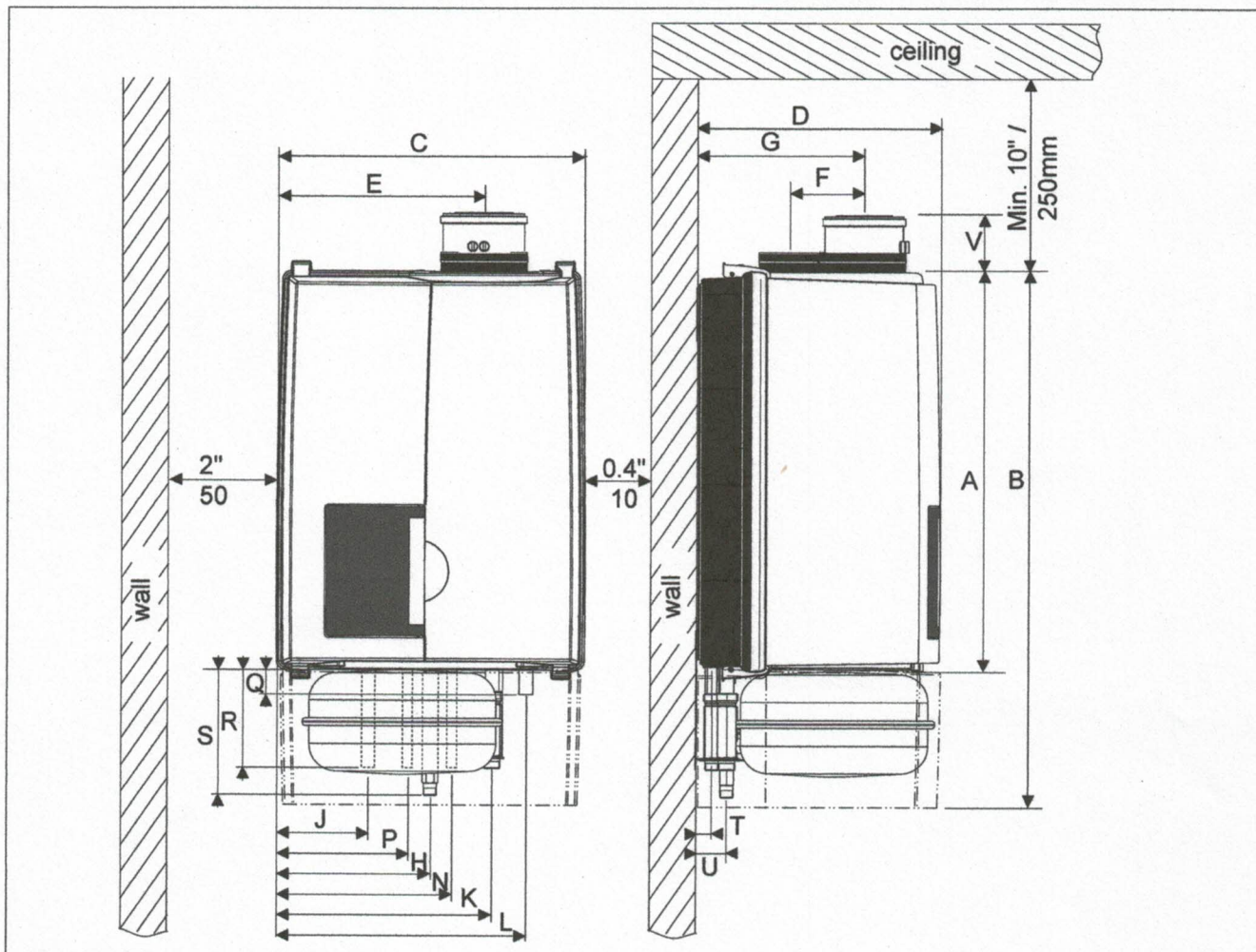
dimensions
