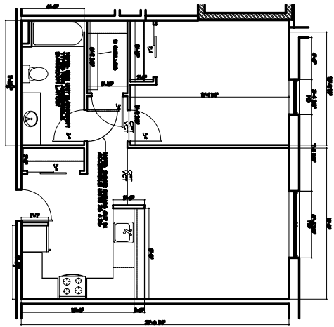
① UNIT TYPE E SCALE: 1/4" = 1'-0"
