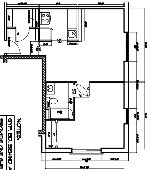
④ UNIT TYPE D SCALE: 1/4" = 1'-0"
