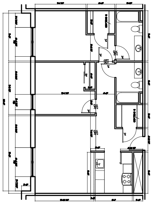
② UNIT TYPE B SCALE: 1/4" = 1'-0"
