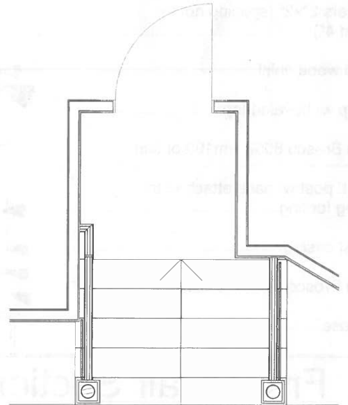
4 Plan SCALE: 1/4" = 1'-0"
