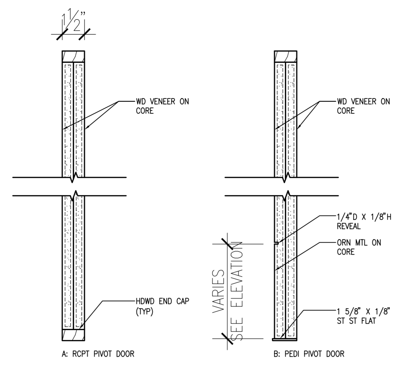
D1 RECEPTION/ PEDI RECEPTION DOOR SECTION SCALE: 3" = 1'-0"
