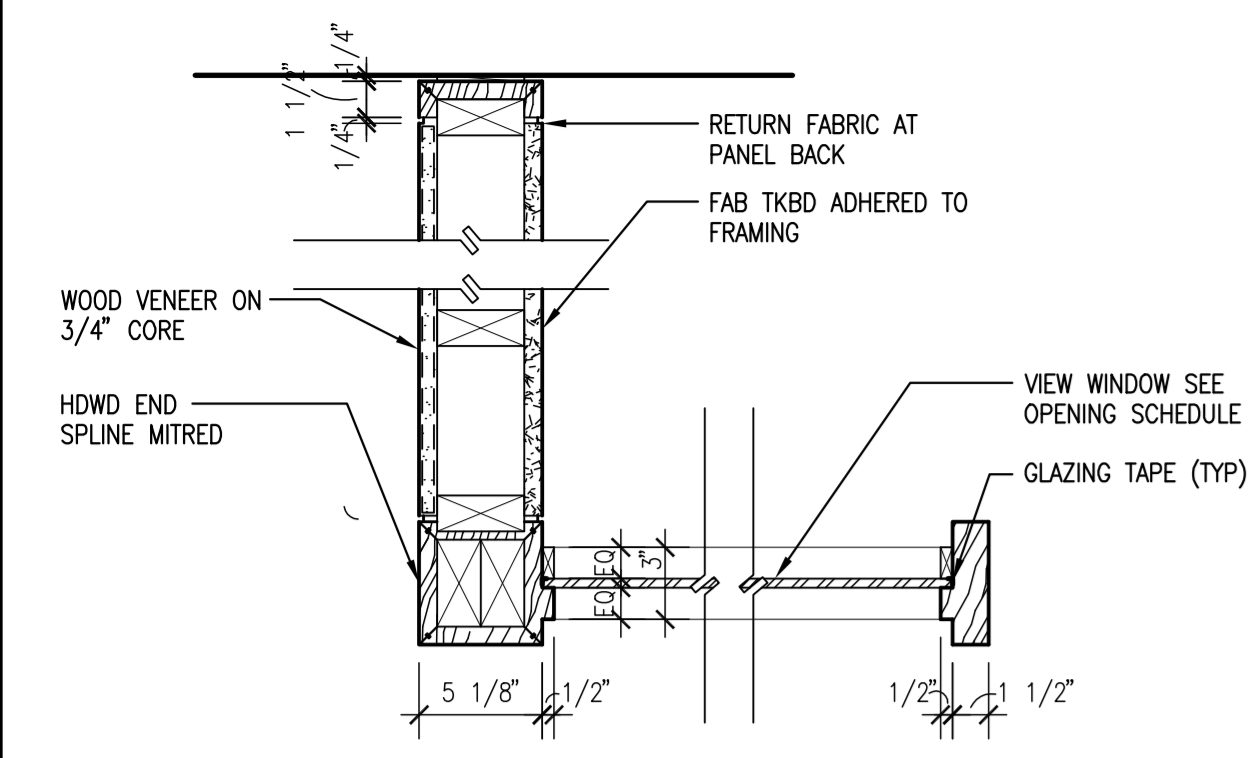
A1 TELEPHONE ALCOVE - PART. PLAN SCALE: 1 1/2" = 1'-0"
