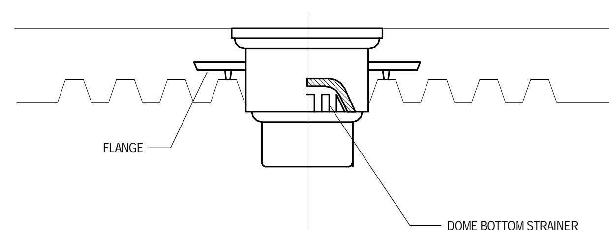
4 GARAGE DRAIN SCALE: 1/8" = 1'-0"
