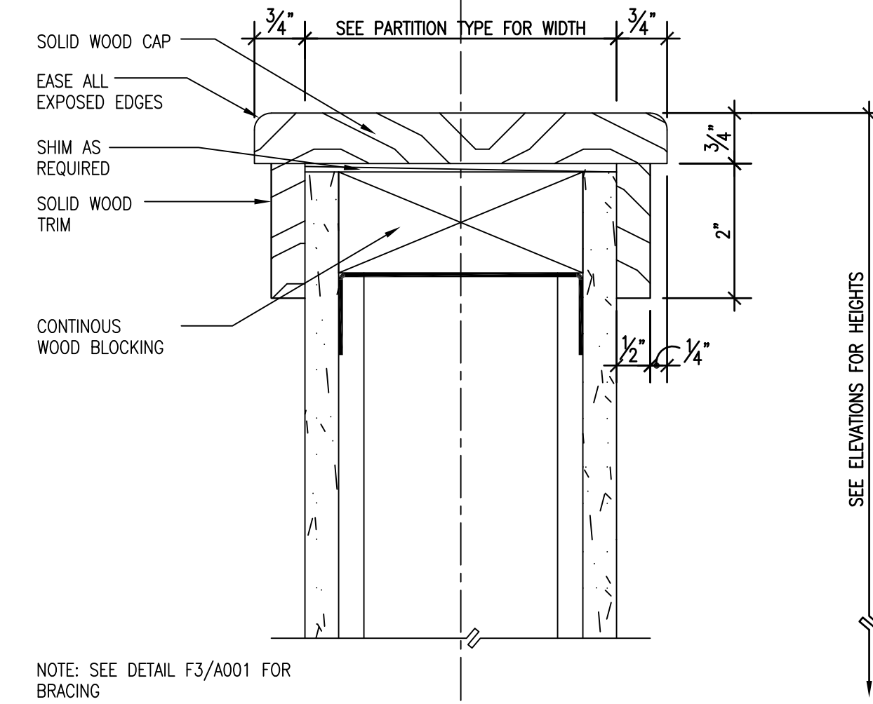
F1 LOW PARTITION WOOD CAP DETAIL SCALE: 6\"/>
