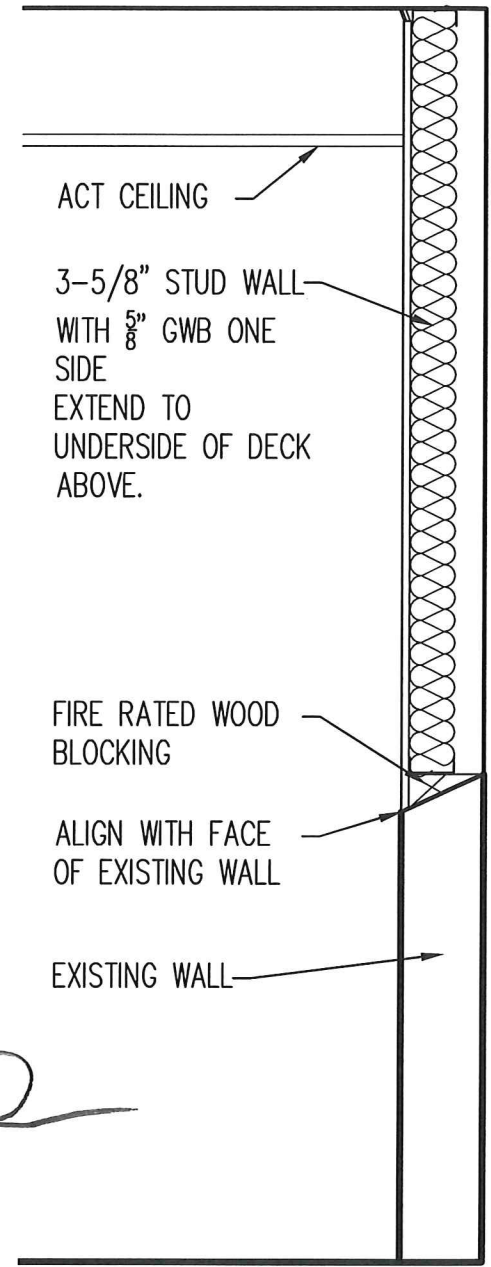
2 WALL SECTION A1.1/A1.3 0 1'-2" SCALE: 3/4" = 1'-0"
