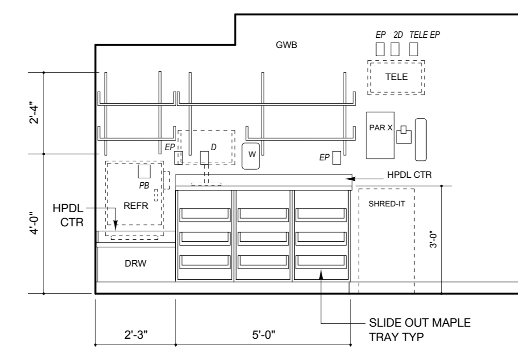
8 MED ROOM ROOM 6145 EAST
