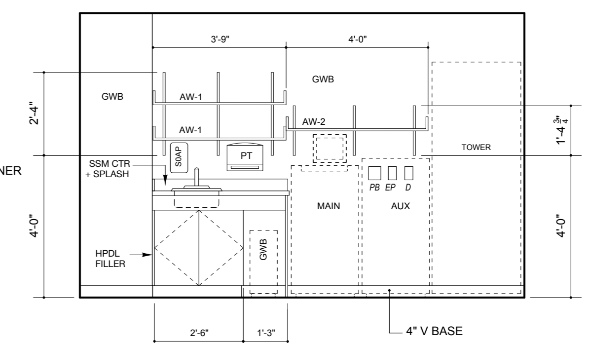
6 MED ROOM ROOM 6145 WEST
