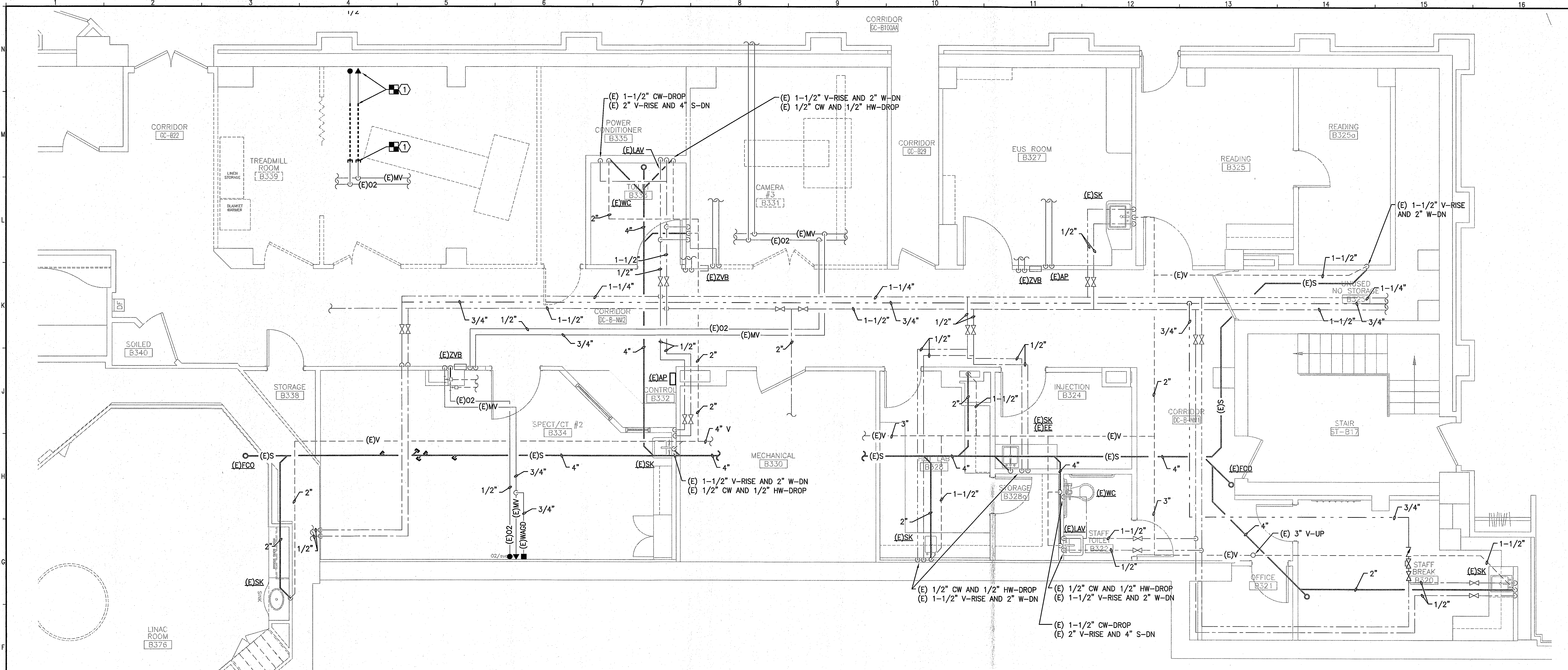
F1 HVAC PIPING DEMOLITION PLAN
