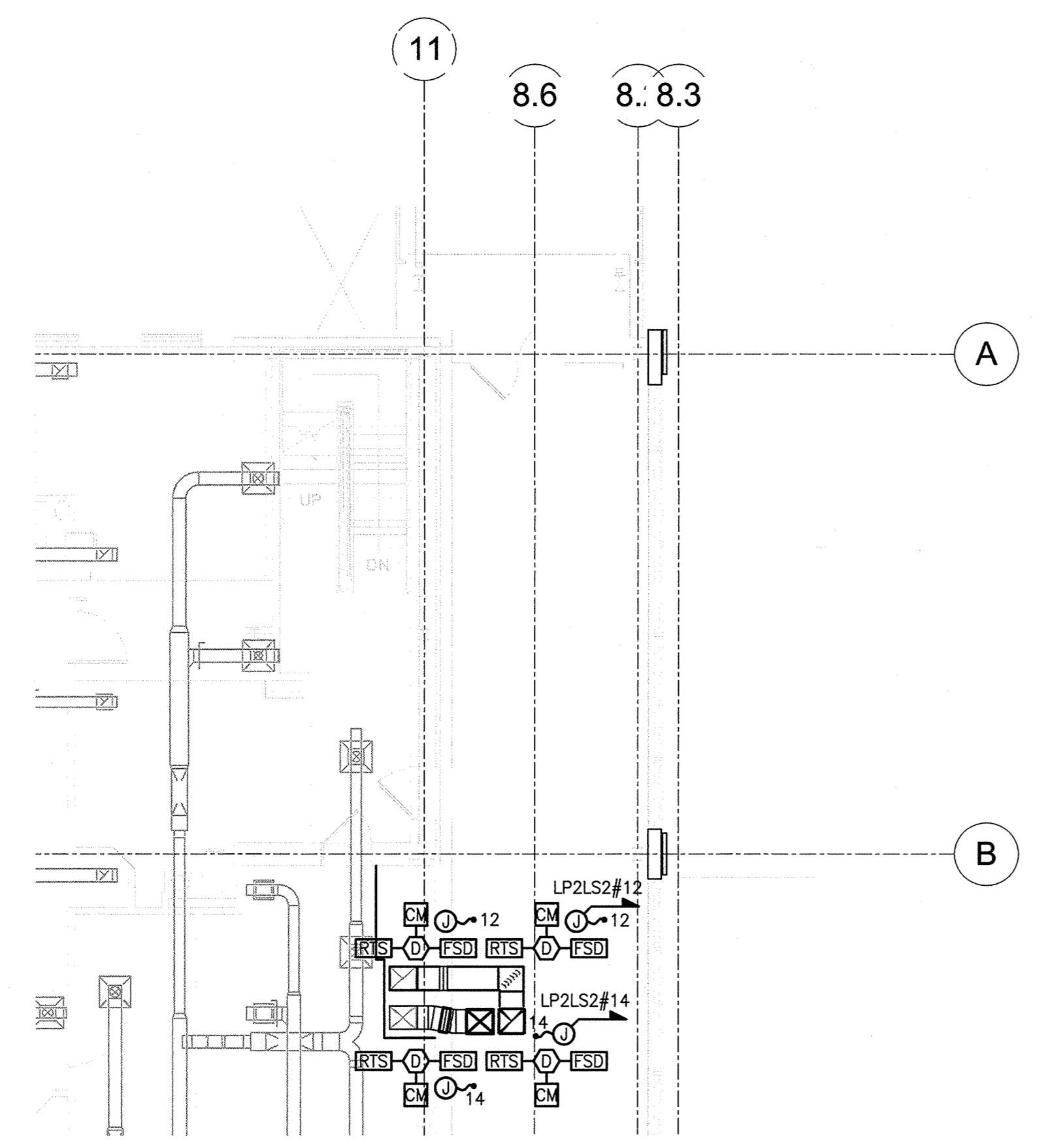
2 FIRE ALARM PART PLAN SCALE: 1/8" = 1'-0"
