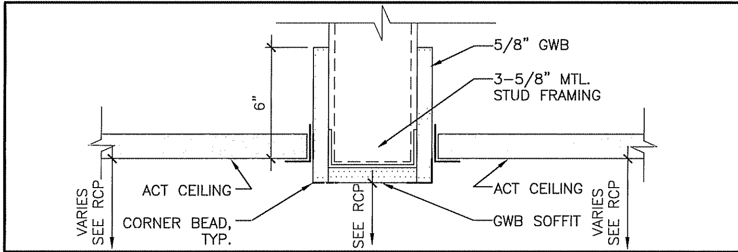
E1 SOFFIT DETAIL
