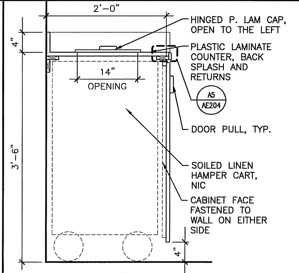
A3 CASEWORK DETAIL
