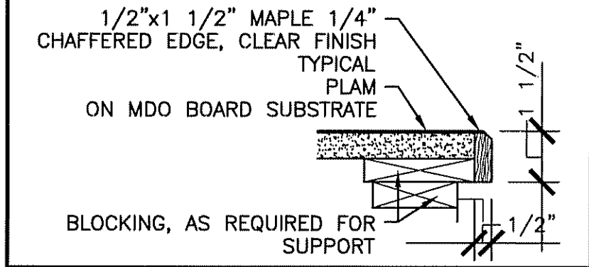
A5 CASEWORK DETAIL
