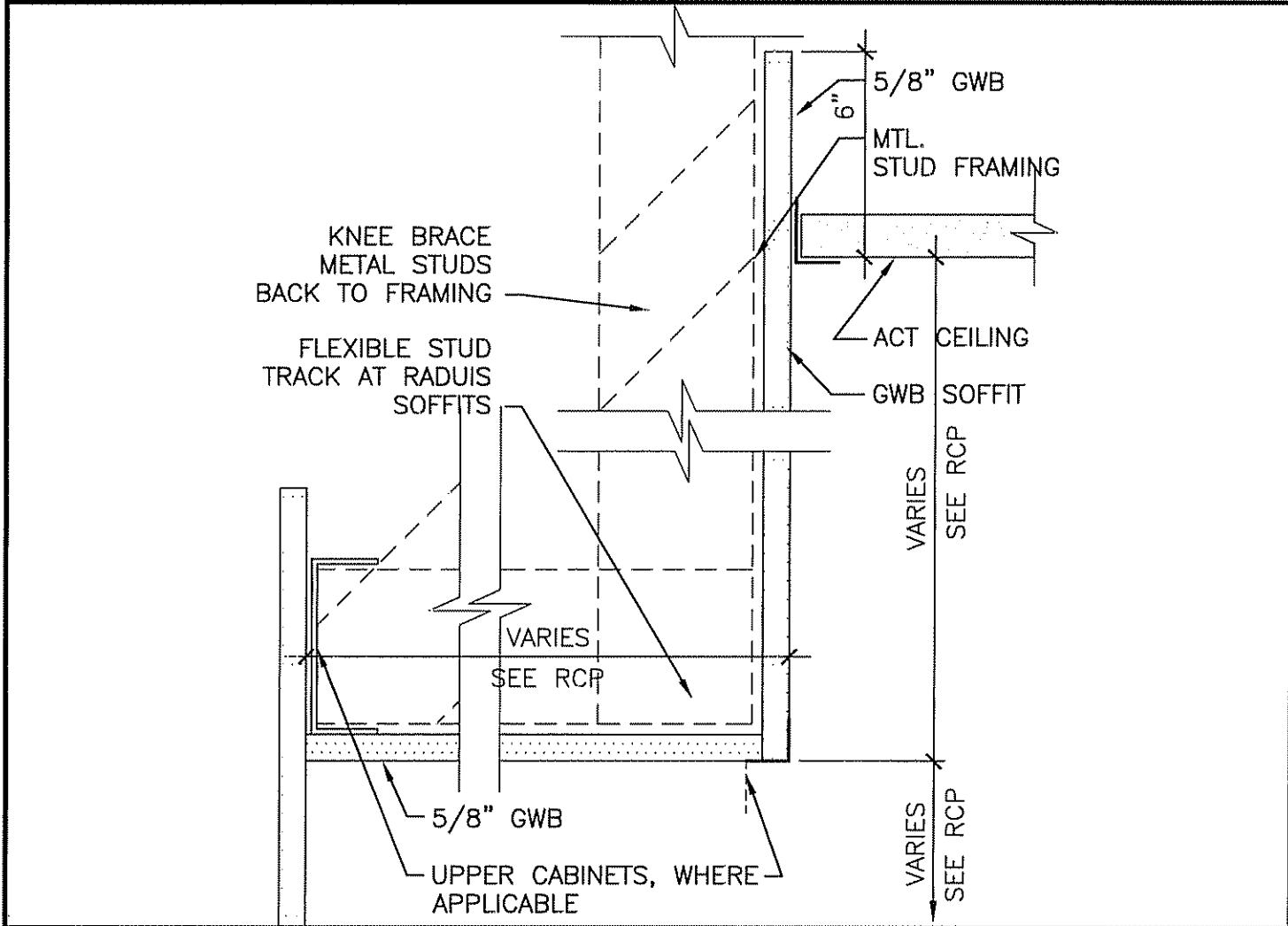
A1 SOFFIT DETAIL
