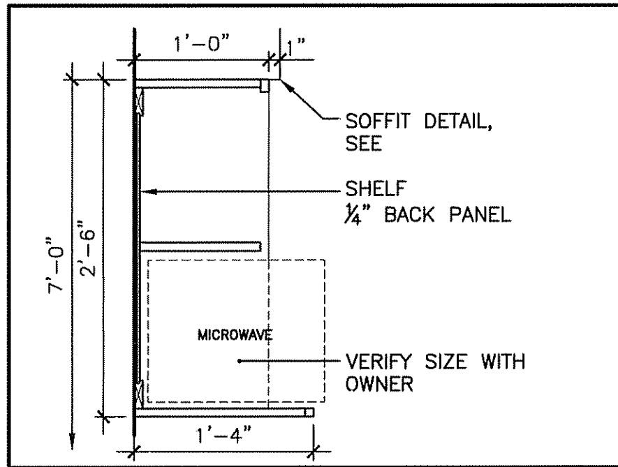
D1 CASEWORK DETAIL
