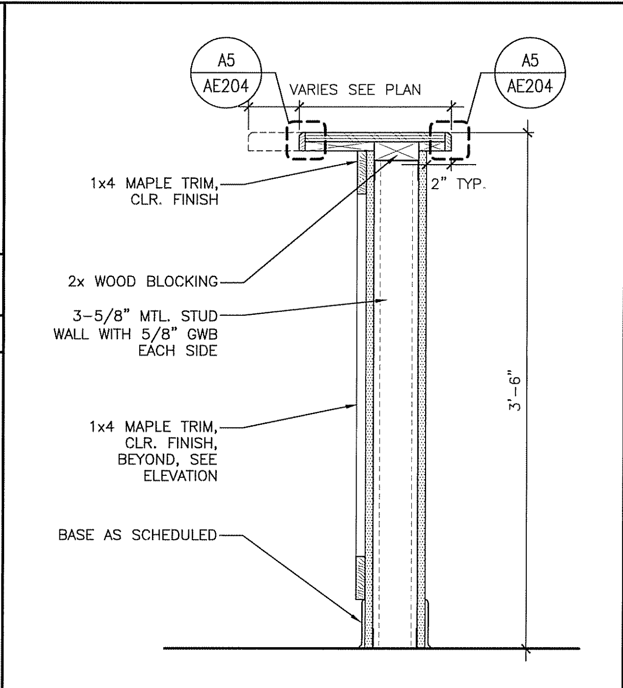
A5 CASEWORK DETAIL
