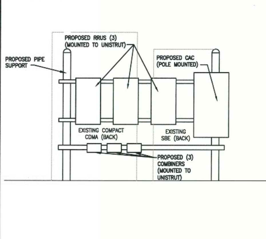
B EQUIPMENT ELEVATION SCALE: N.T.S.
