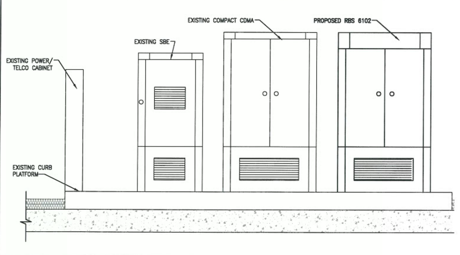
A EQUIPMENT ELEVATION SCALE: N.T.S.
