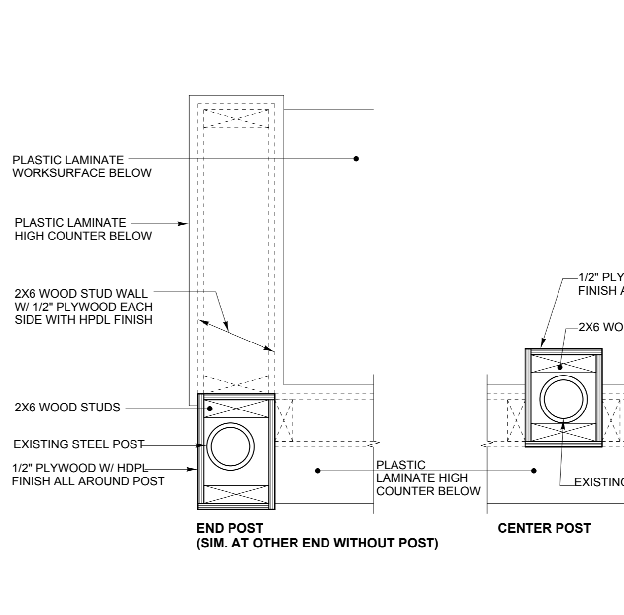
D PLAN DETAIL AT MED ASSIST. 109 SCALE: 1 1/2" = 1'-0"
