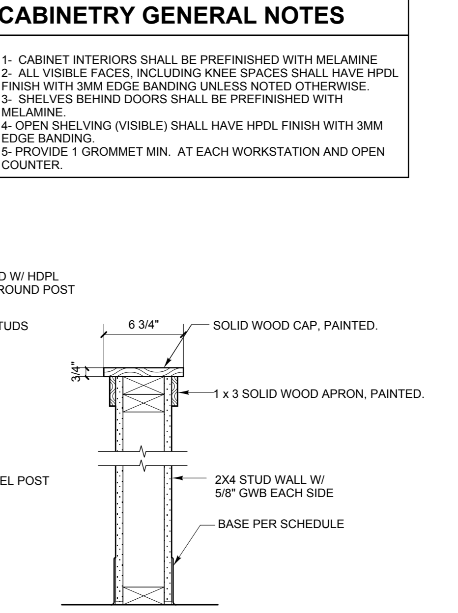
E KNEE WALL DETAIL SCALE: 1 1/2" = 1'-0"
