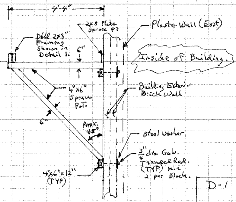
Elevation C-C Scale: 1" = 1'
