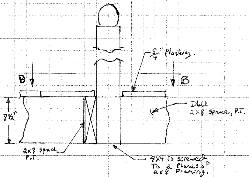
Detail A - Elev Scale: 2" = 1'
