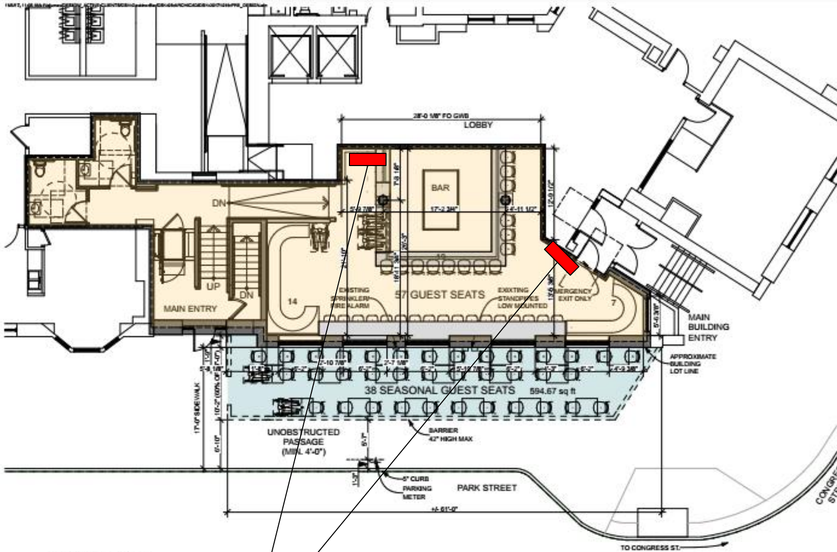
1 MAIN LEVEL SCALE: 1/8" = 1'-0"
