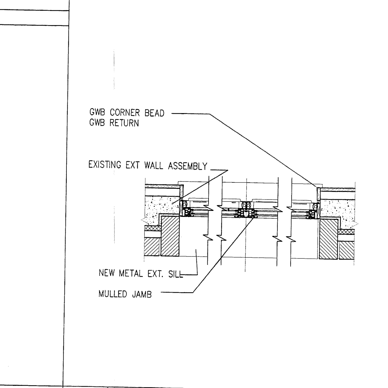
A5 SILL DETAIL 3/4"=1'-0"
