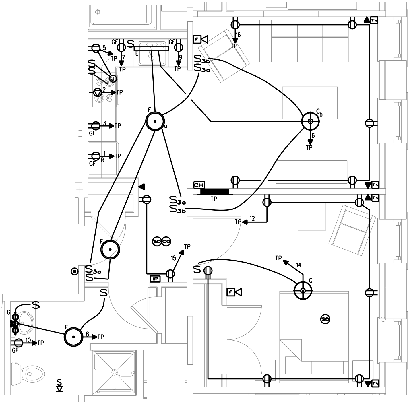
UNIT 310 1B-7 SCALE: 1/4" = 1'-0"
