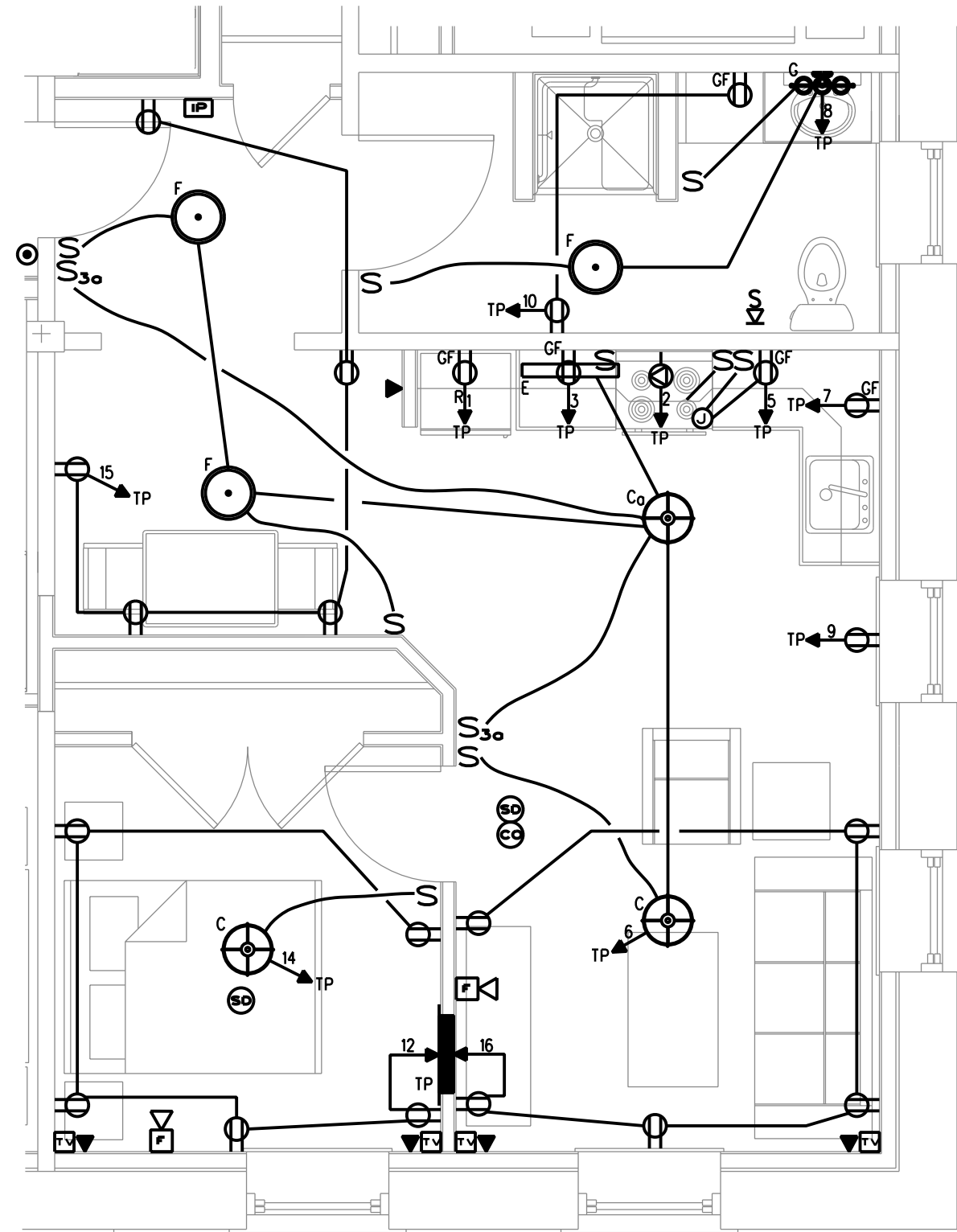
UNIT 311 1B-8 SCALE: 1/4" = 1'-0"
