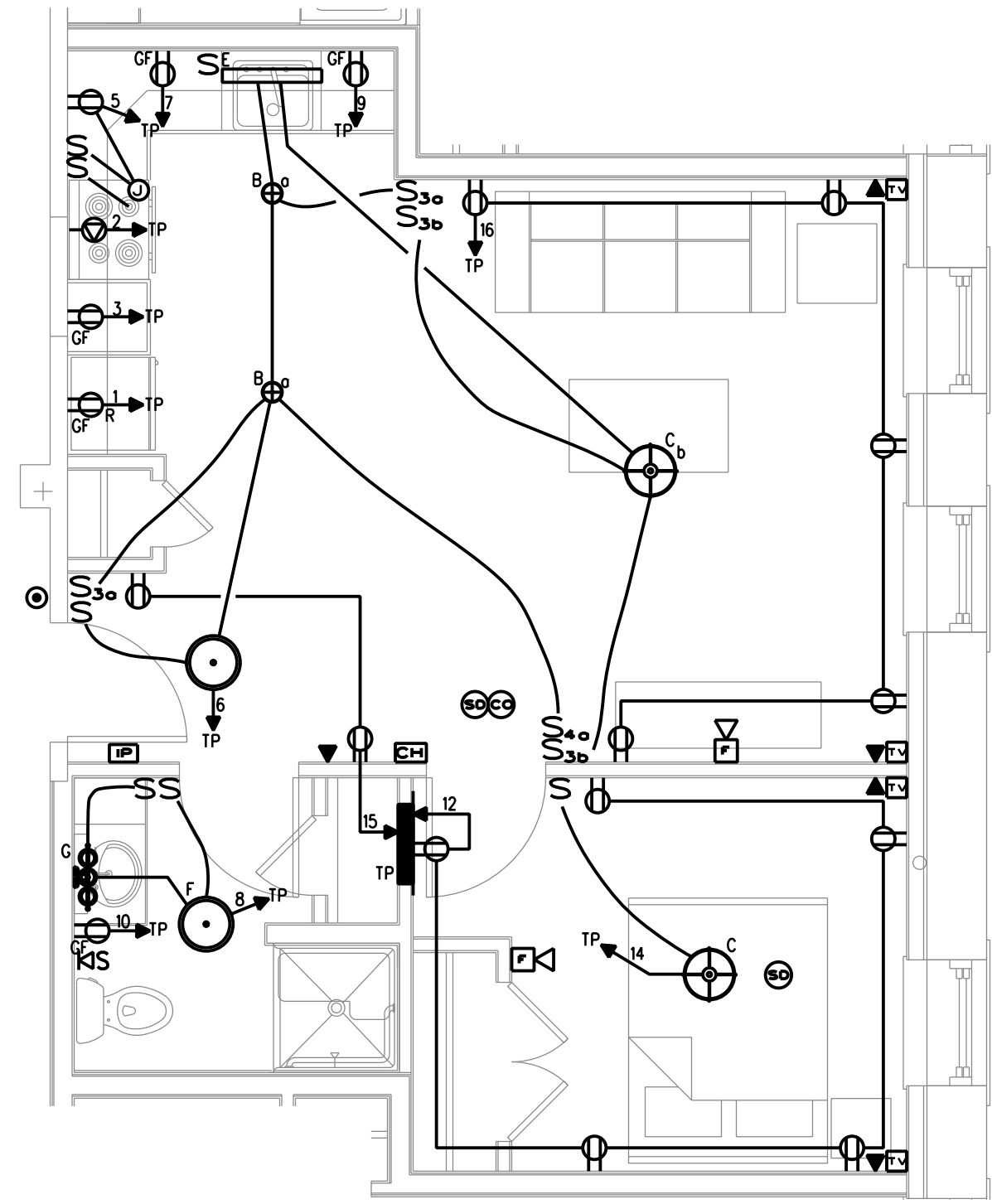
UNIT 210 1B-6 SCALE: 1/4" = 1'-0"
