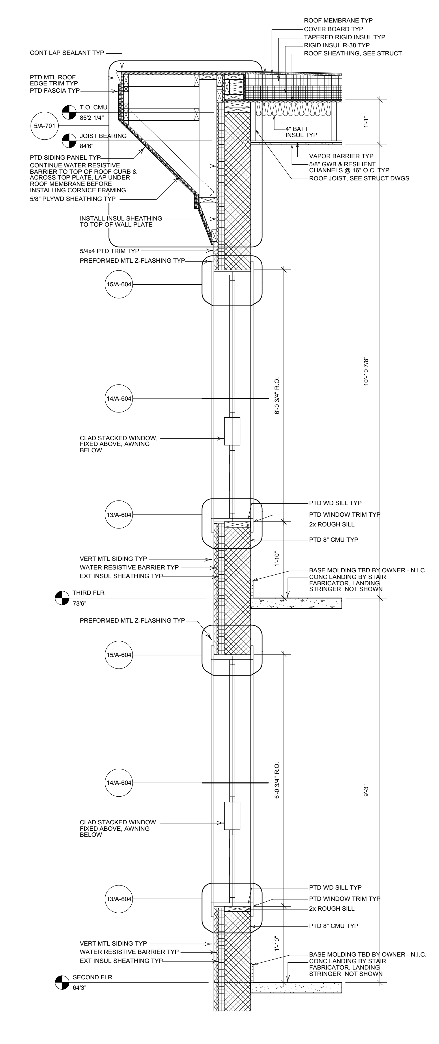
2 WALL SECTION @ STAIR CONT A-802 Scale: 3/4" = 1'-0"
