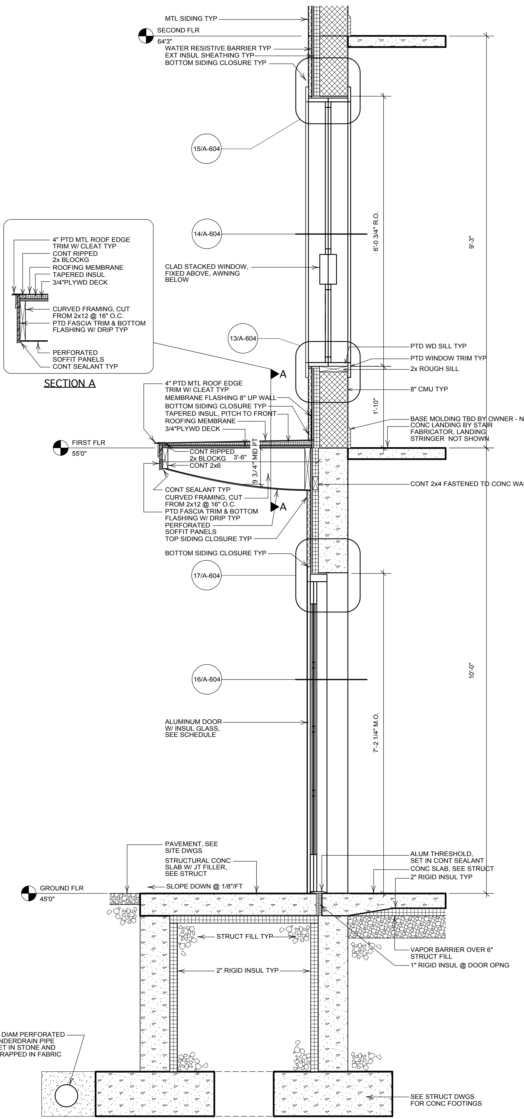
2 WALL SECTION @ STAIR A-802 Scale: 3/4" = 1'-0"
