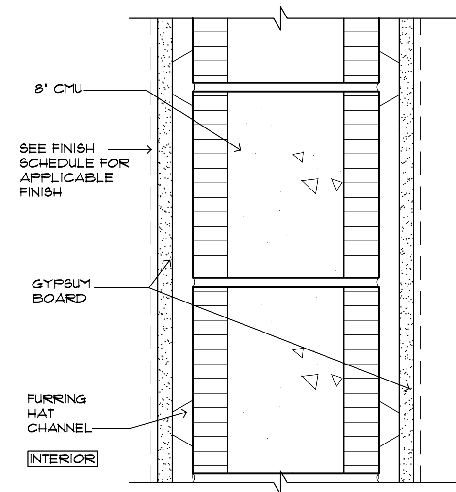
M-4 2 HR. FIRE RATING UL-U905
