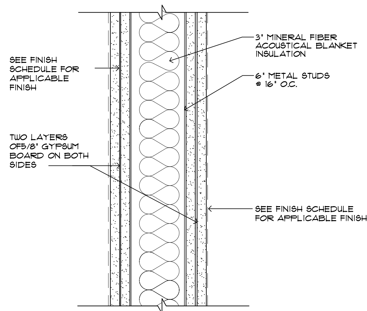
P-1-A 2 HR. FIRE RATING UL-U419
