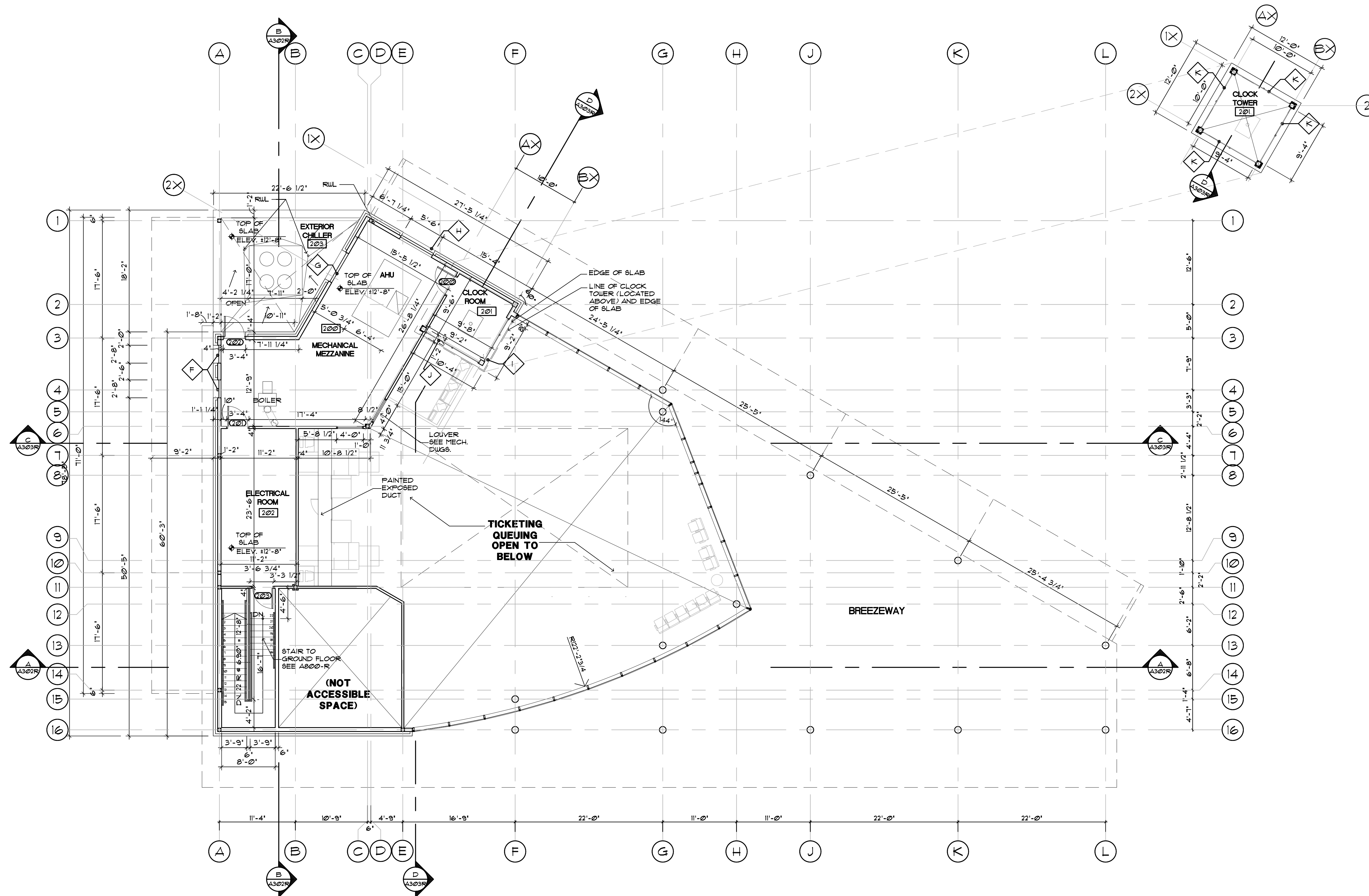
MEZZANINE FLOOR PLAN SCALE: 1/8" = 1'-0"
