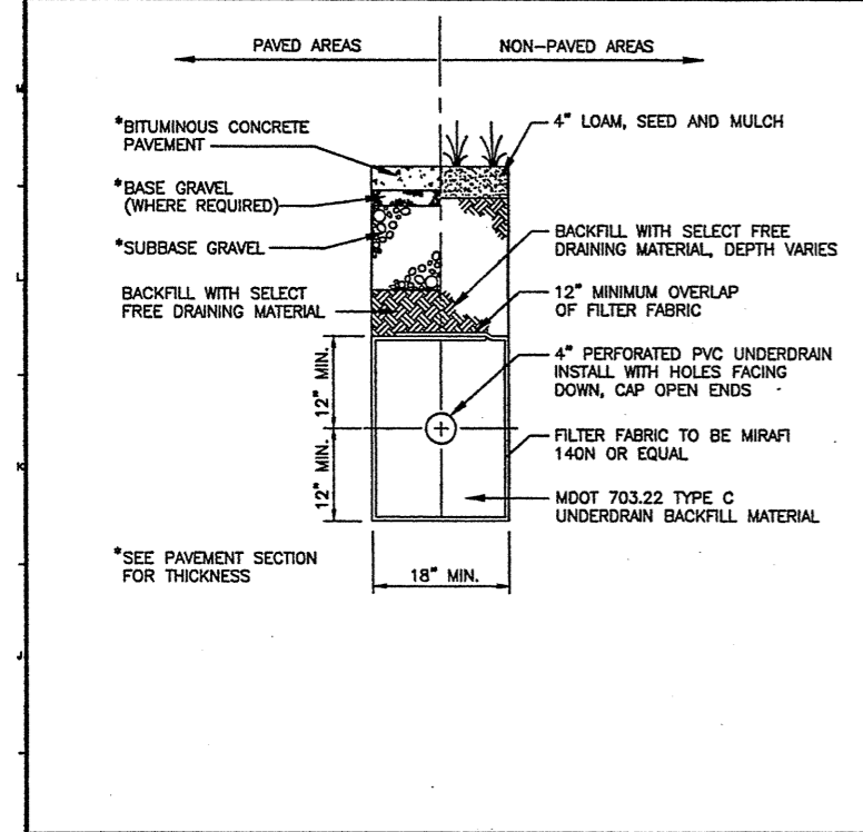
E1 GRANITE CURB DETAIL N.T.S.
