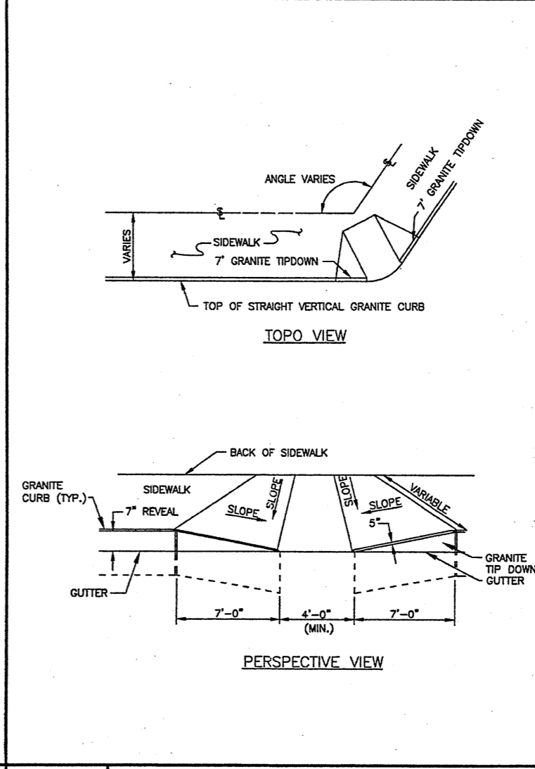
A14 PEDESTRIAN RAMP N.T.S.
