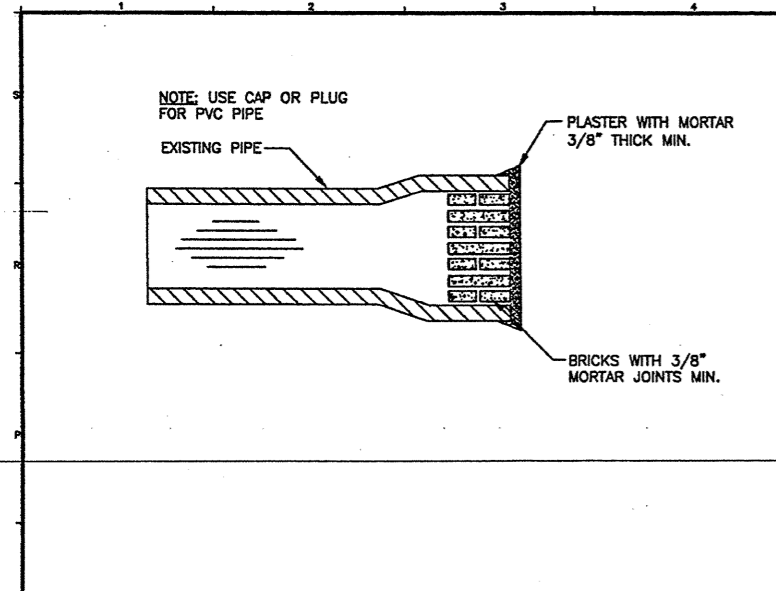
N1 MASONRY PLUG DETAIL N.T.S.
