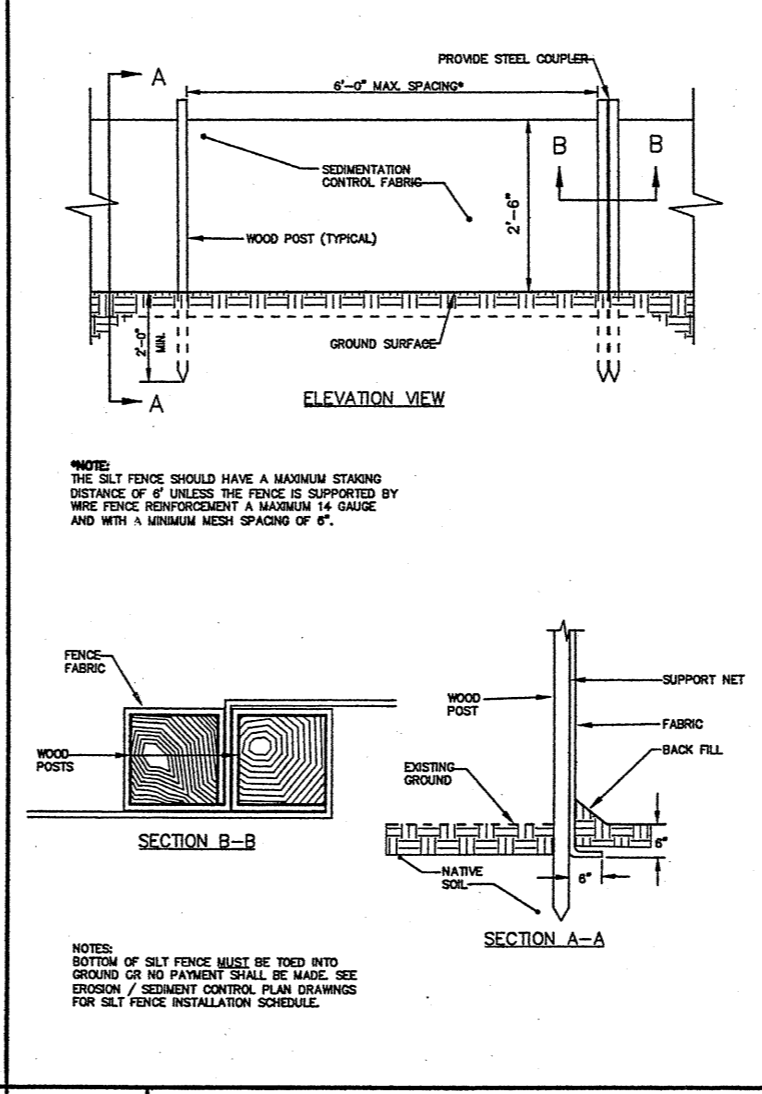
A10 SILTATION FENCE DETAIL N.T.S.
