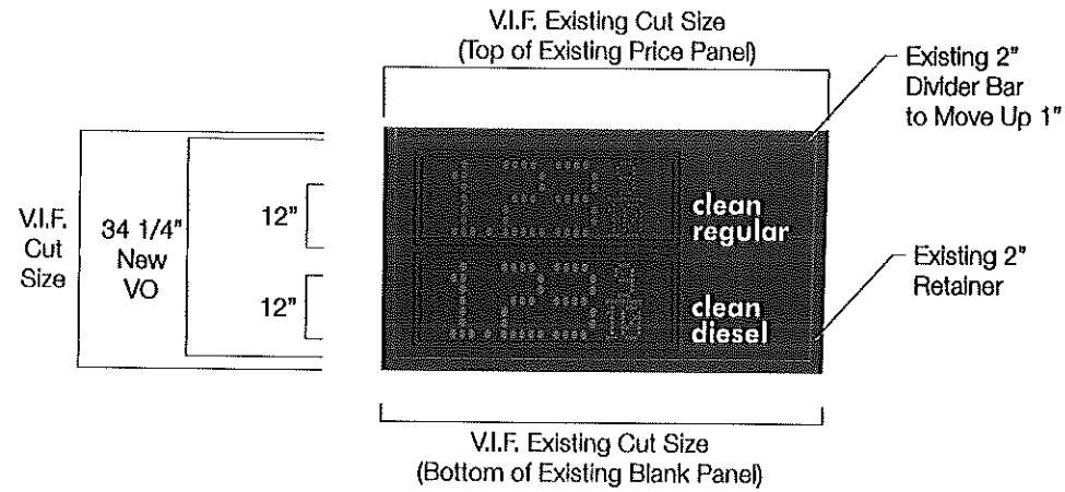
A Sign Elevation Scale: 3/8"=1'-0"
