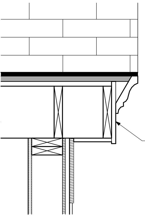
5 DETAIL - RAKE SCALE: 1 1/2" = 1'-0"
