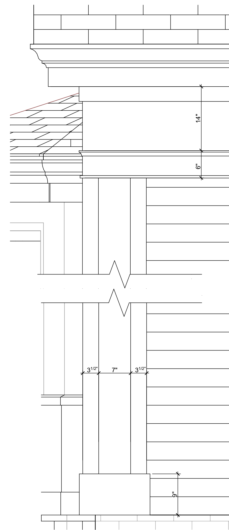
1 CORNER ELEVATION SCALE: 1" = 1'-0"
