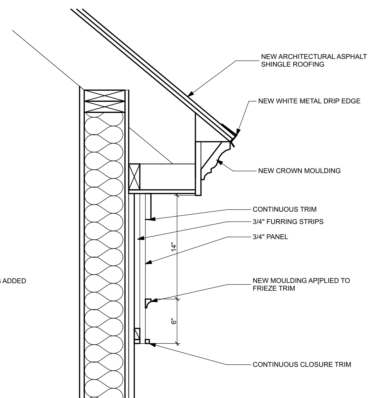
6 DETAIL - EAVE SCALE: 1 1/2" = 1'-0"
