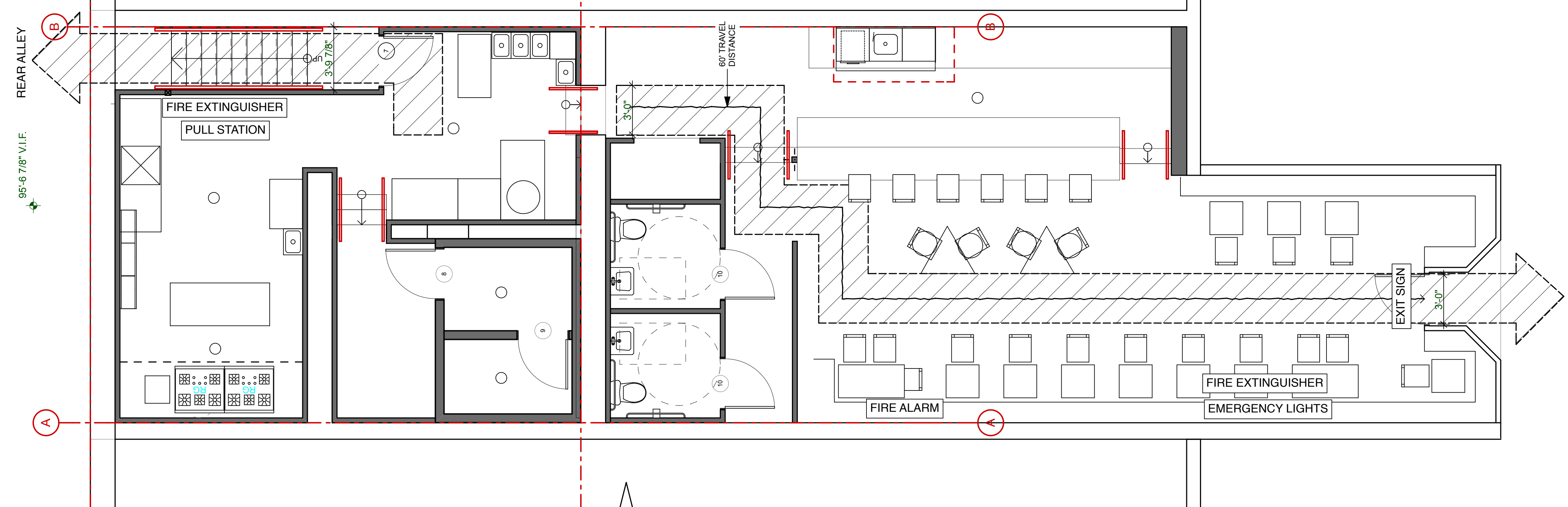
1 LIFE SAFETY SCALE: 1/4" = 1'-0"
