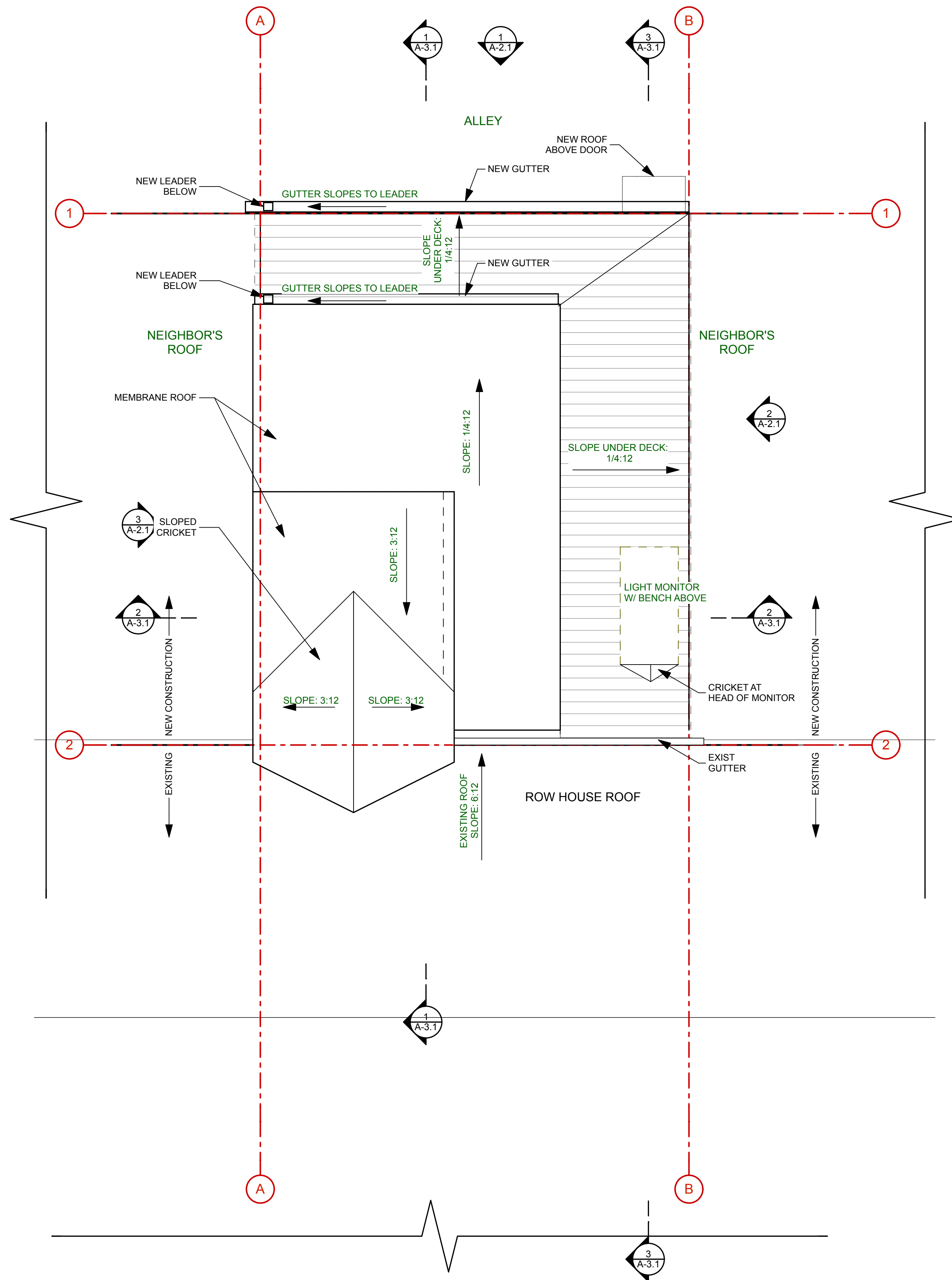
2 ROOF SCALE: 1/4" = 1'-0"
