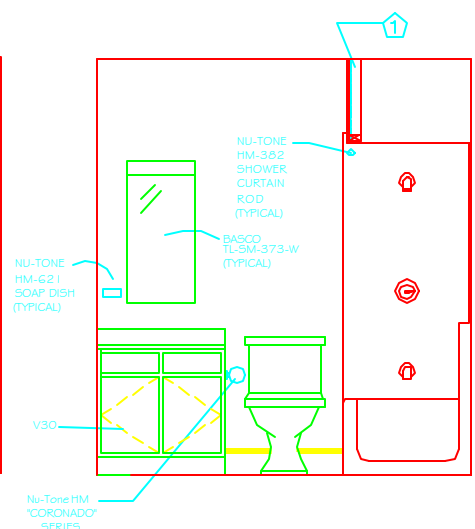
TOILET ELEV.
