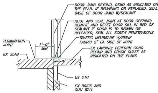
DOOR SILL
