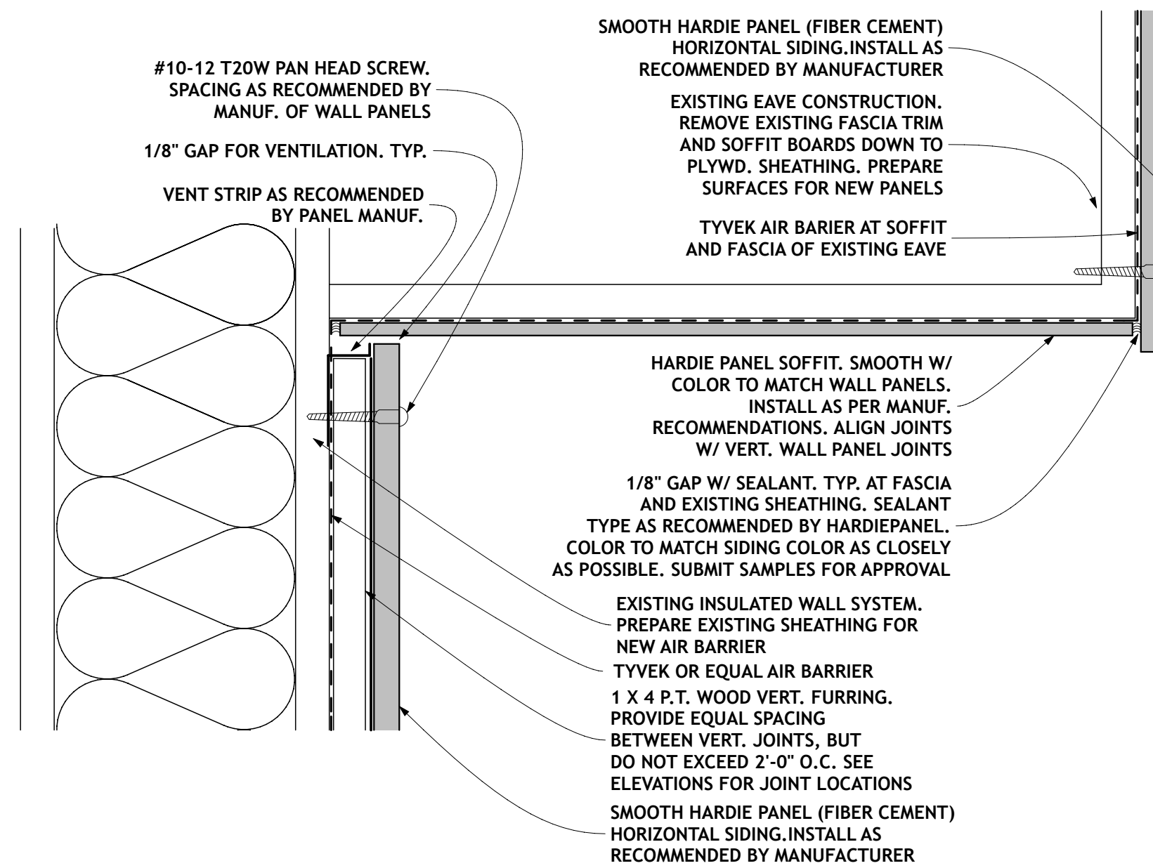
2 SECTION DETAIL- EXISTING SOFFIT SCALE: 6" = 1'-0"
