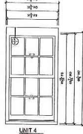
UNIT 4 SCALE: 3/4\"/>
