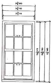
UNIT 2 SCALE: 3/4\"/>
