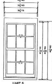
UNIT 5 SCALE: 3/4\"/>
