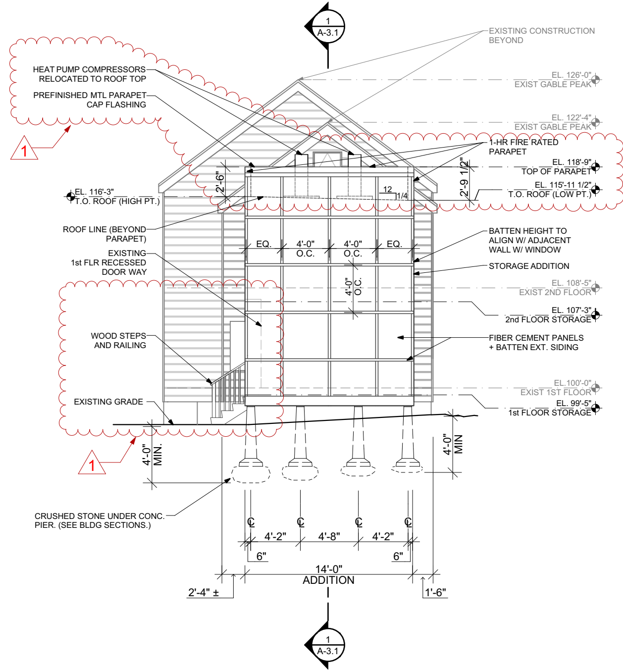
1 EAST ELEVATION SCALE: 1/8" = 1'-0"
