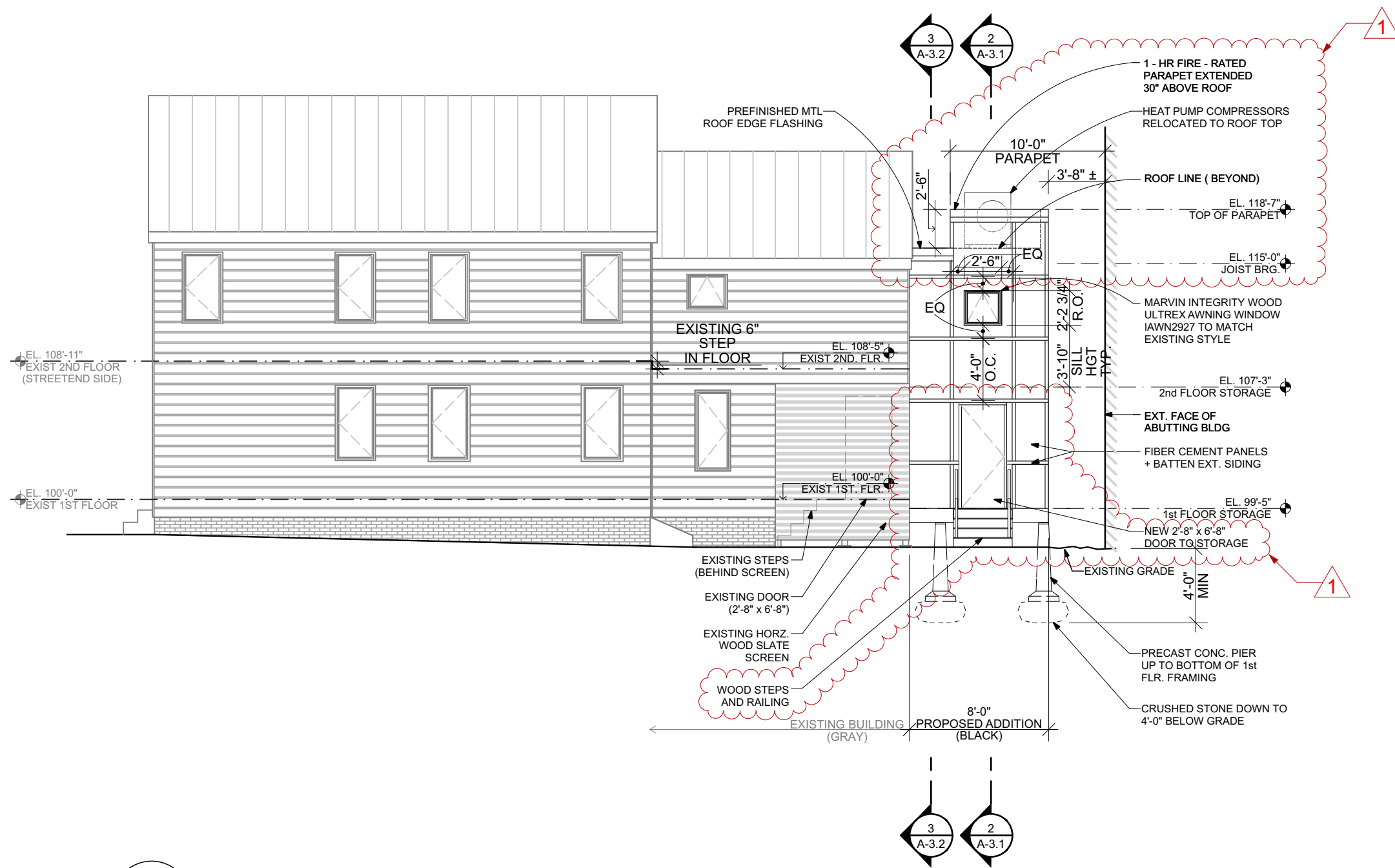
1 SOUTH ELEVATION A-2.2 SCALE: 1/8" = 1'-0"
