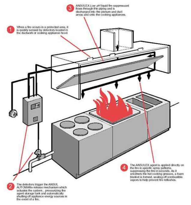
Typ. Exhaust Hood Scale: N.T.S.
