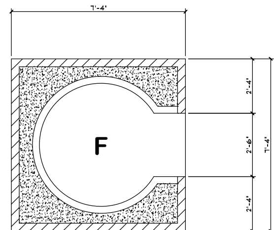
Typ. Ansul System Scale: N.T.S.
