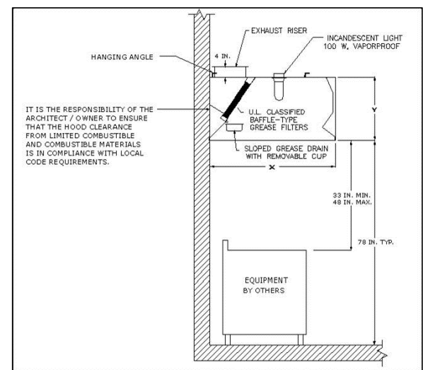
Typ. Ansul System Scale: N.T.S.
