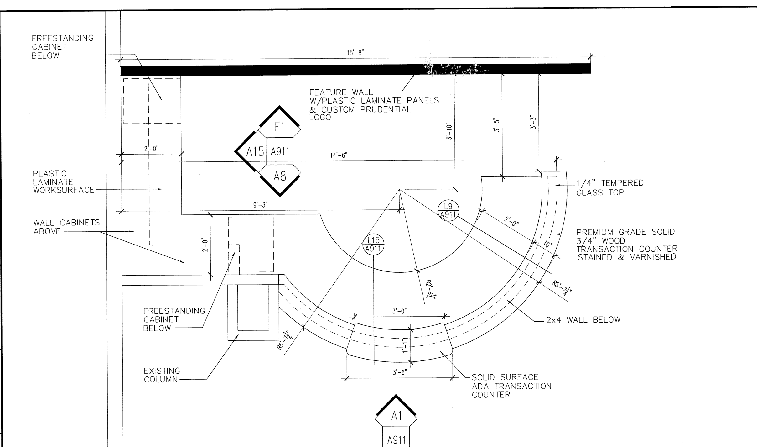
L1 RECEPTION 429 1/2\"/>
