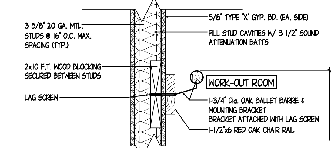
8 DETAIL SCALE: 1-1/2" = 1'-0"
