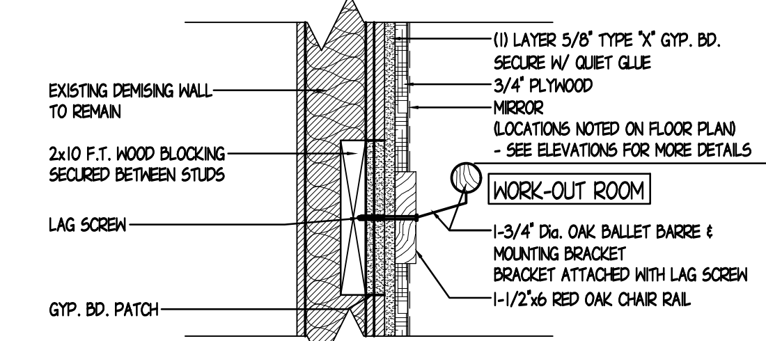
2 DETAIL SCALE: 1-1/2" = 1'-0"
