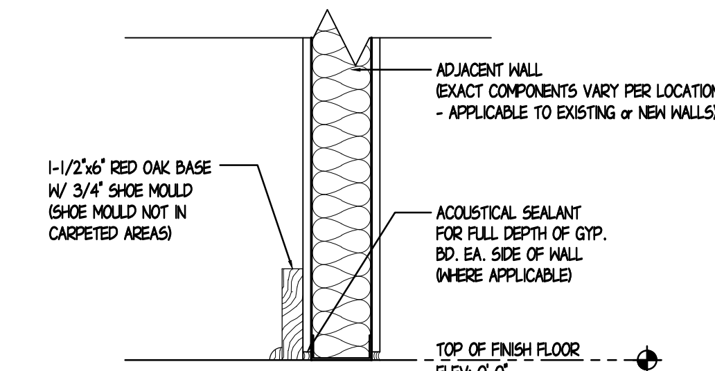
10 DETAIL SCALE: 1-1/2" = 1'-0"
