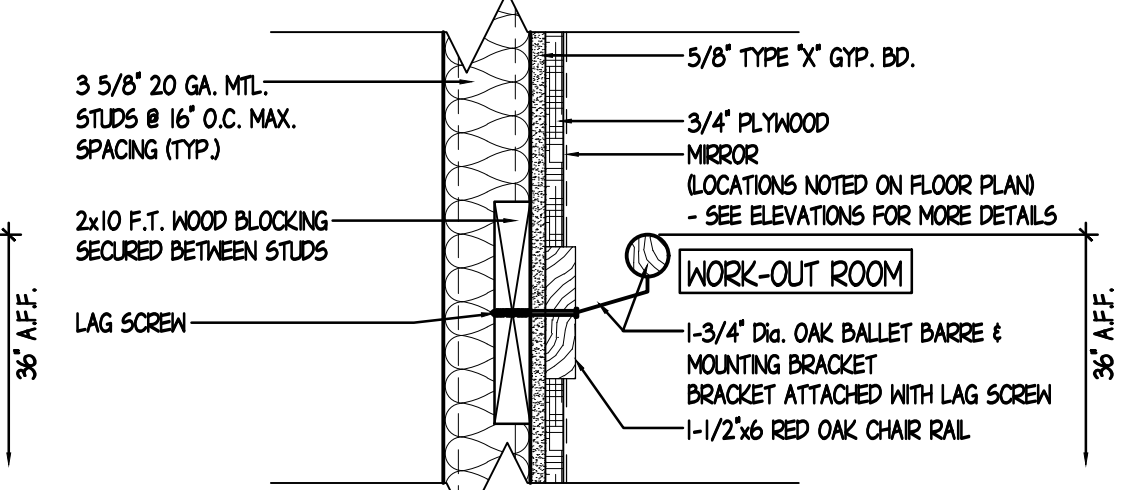
5 DETAIL SCALE: 1-1/2" = 1'-0"
