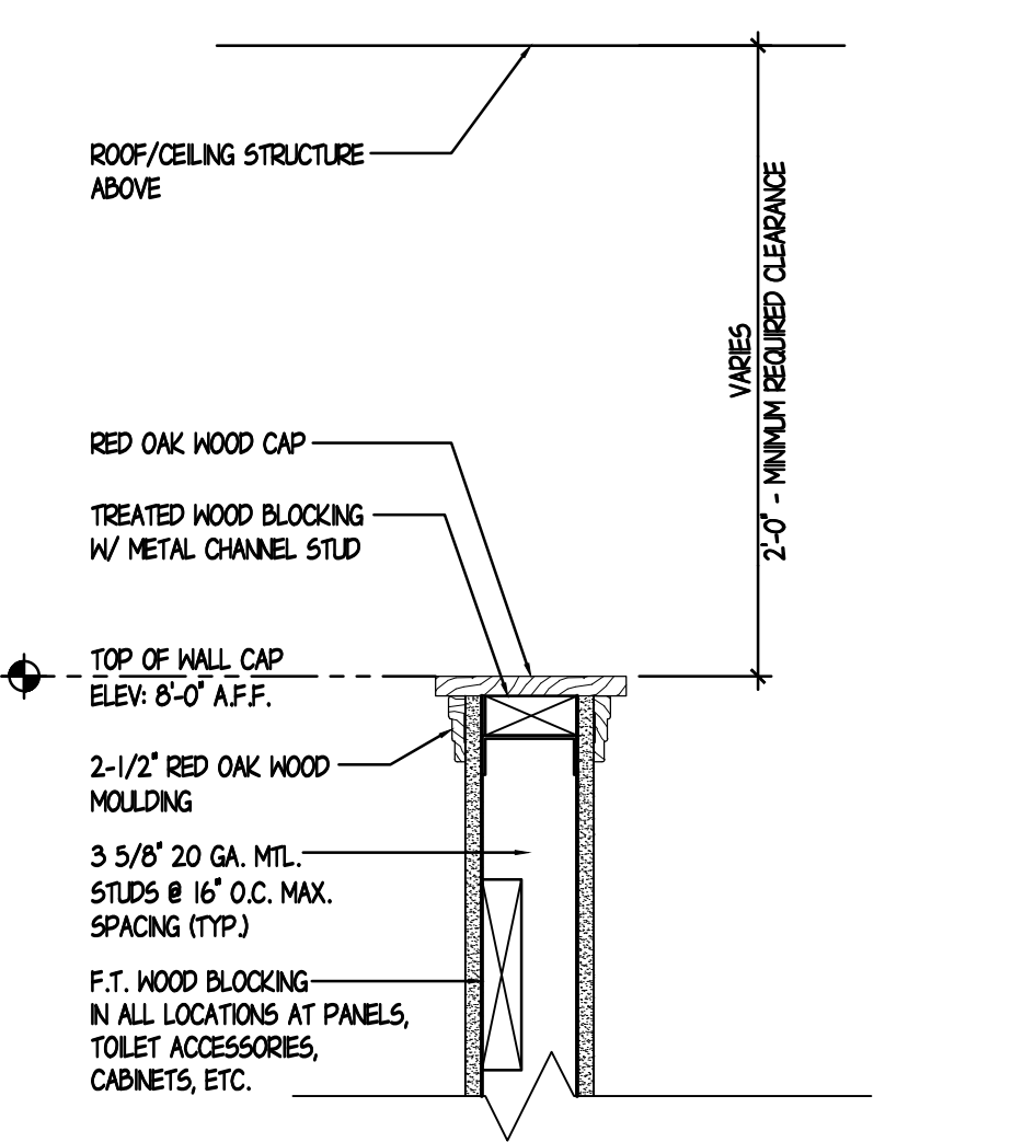
11 WALL CAP DETAIL SCALE: 1-1/2" = 1'-0"
