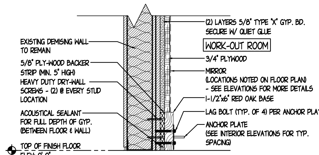
1 DETAIL SCALE: 1-1/2" = 1'-0"
