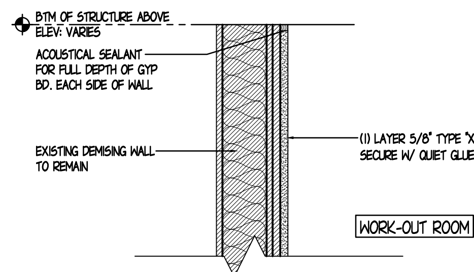
3 DETAIL SCALE: 1-1/2" = 1'-0"
