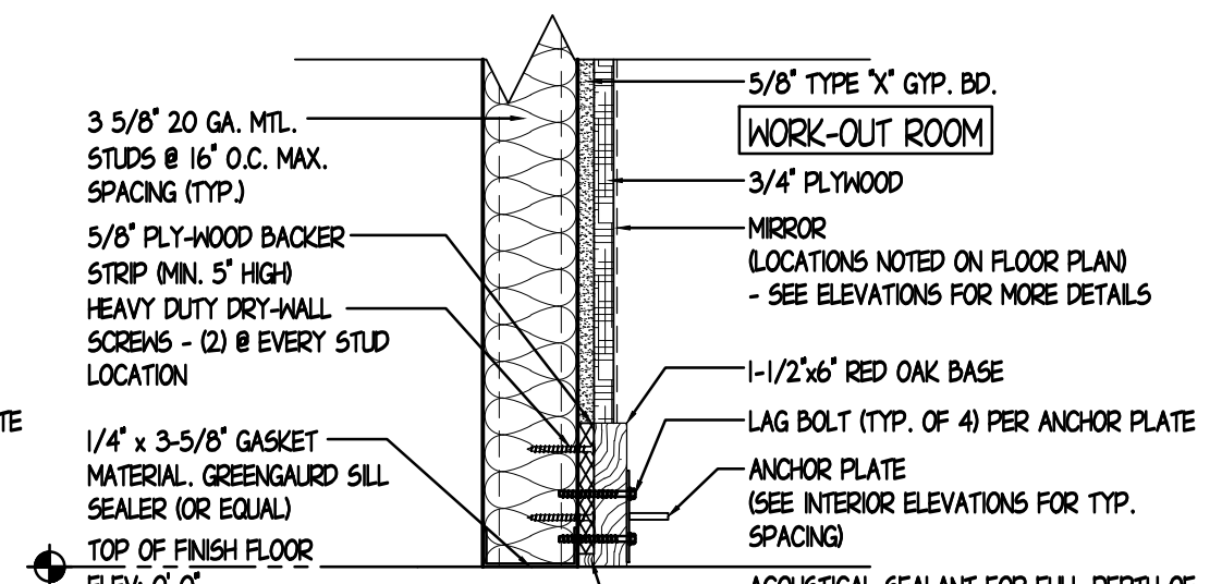
4 DETAIL SCALE: 1-1/2" = 1'-0"
