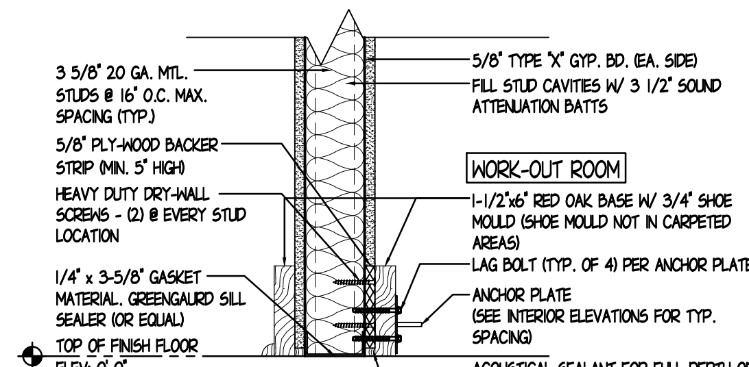
7 DETAIL SCALE: 1-1/2" = 1'-0"
