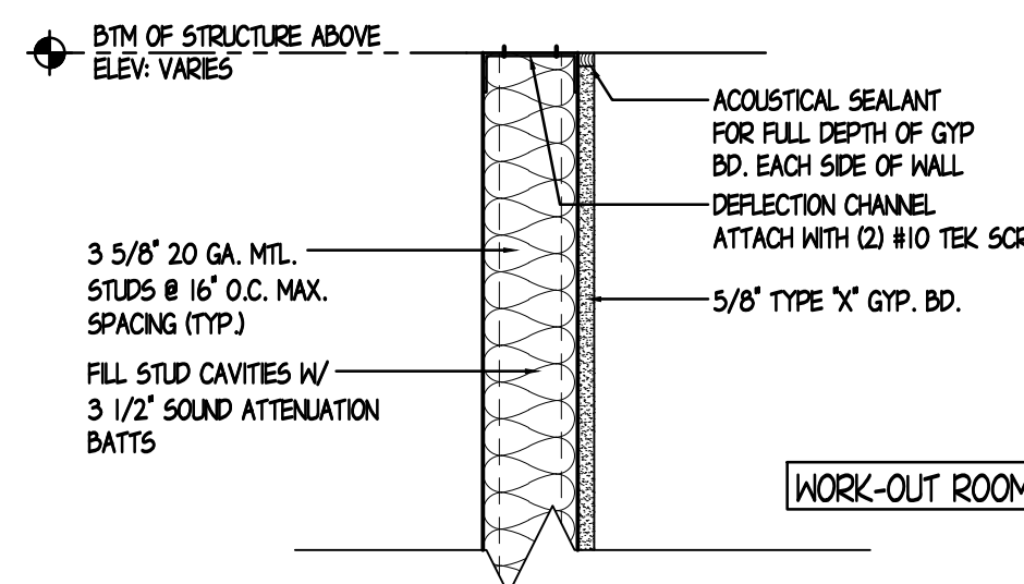
6 DETAIL SCALE: 1-1/2" = 1'-0"
