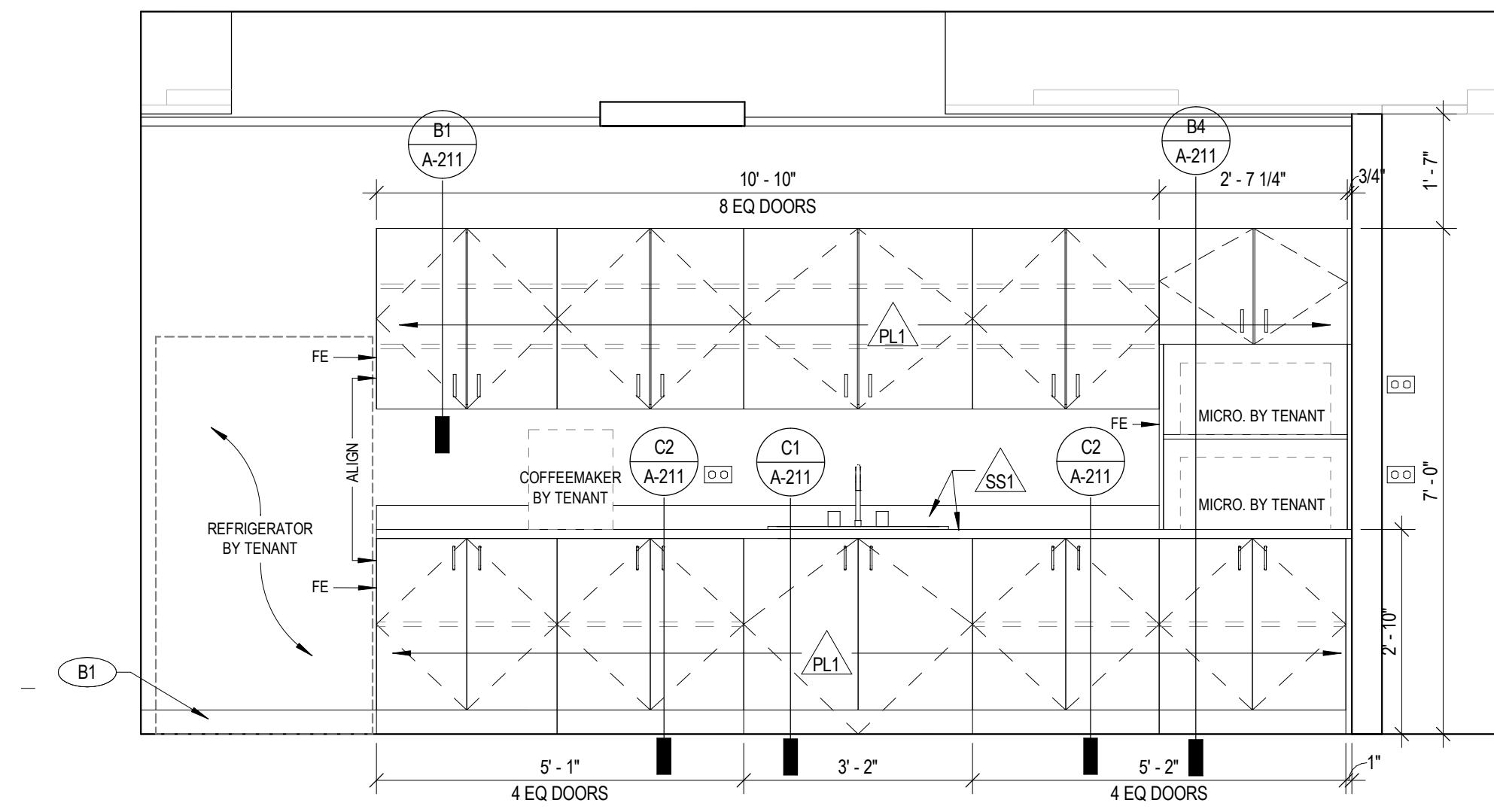
D1 ELEVATION @ PANTRY 503 SCALE: 1/2" = 1'-0"
