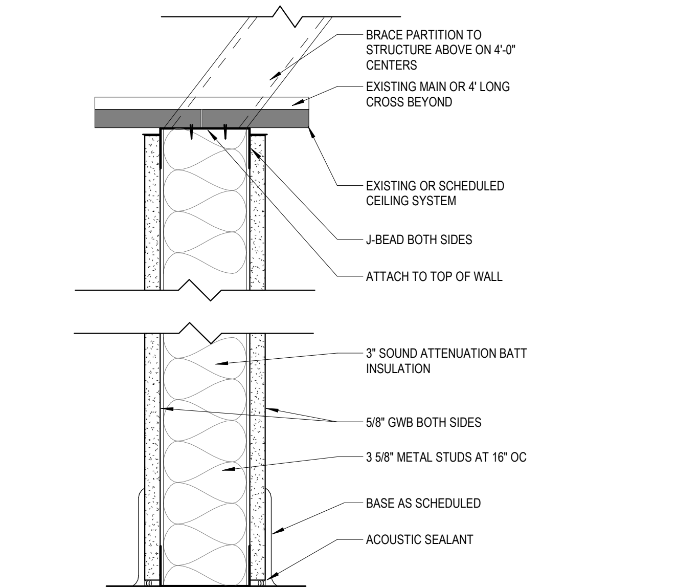
A1 TYPE 1 - TO CLG. (3 5/8") SCALE: 3" = 1'-0"
