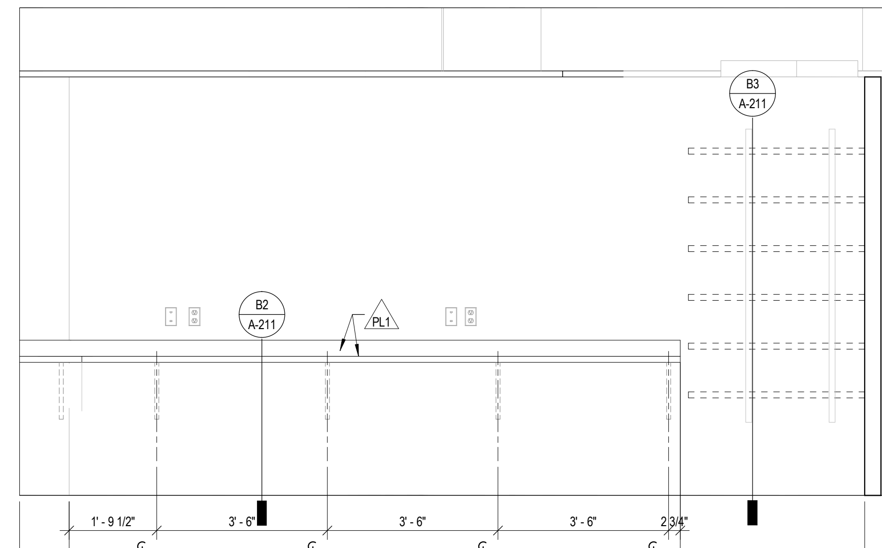
D2 ELEVATION @ IT ROOM 509 SCALE: 1/2" = 1'-0"
