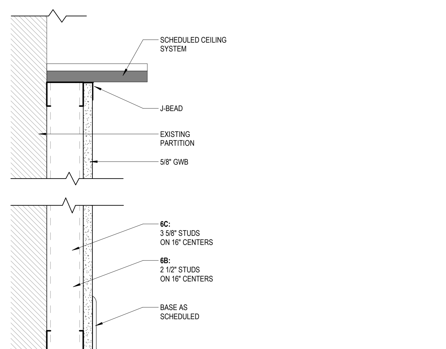
A2 TYPE 6 - FURRING TO CLG. SCALE: 3" = 1'-0"
