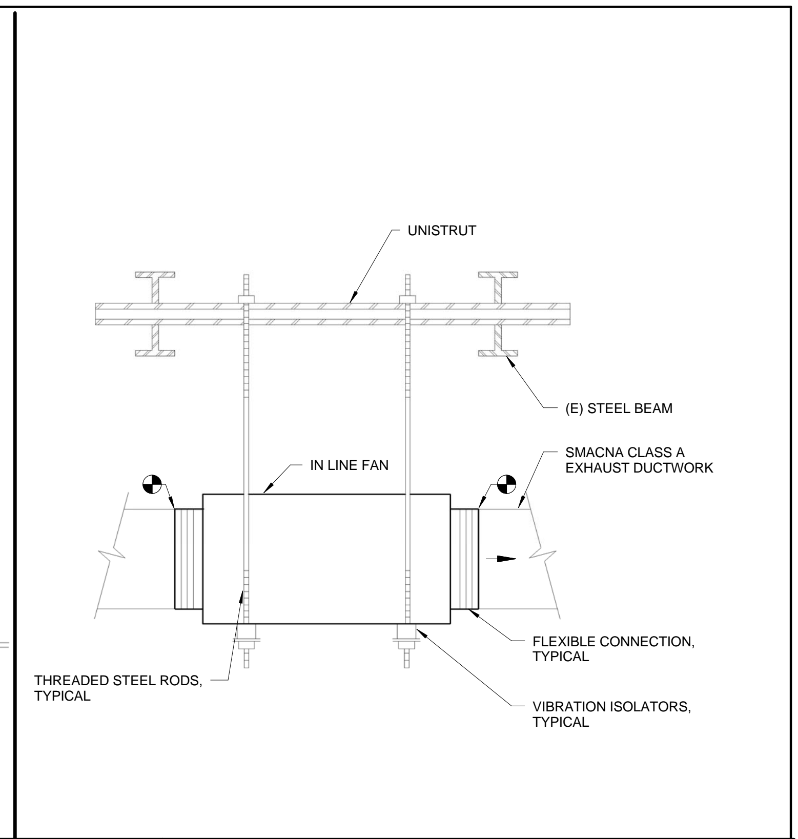
E8 DETAIL - IN LINE EXHAUST FAN
