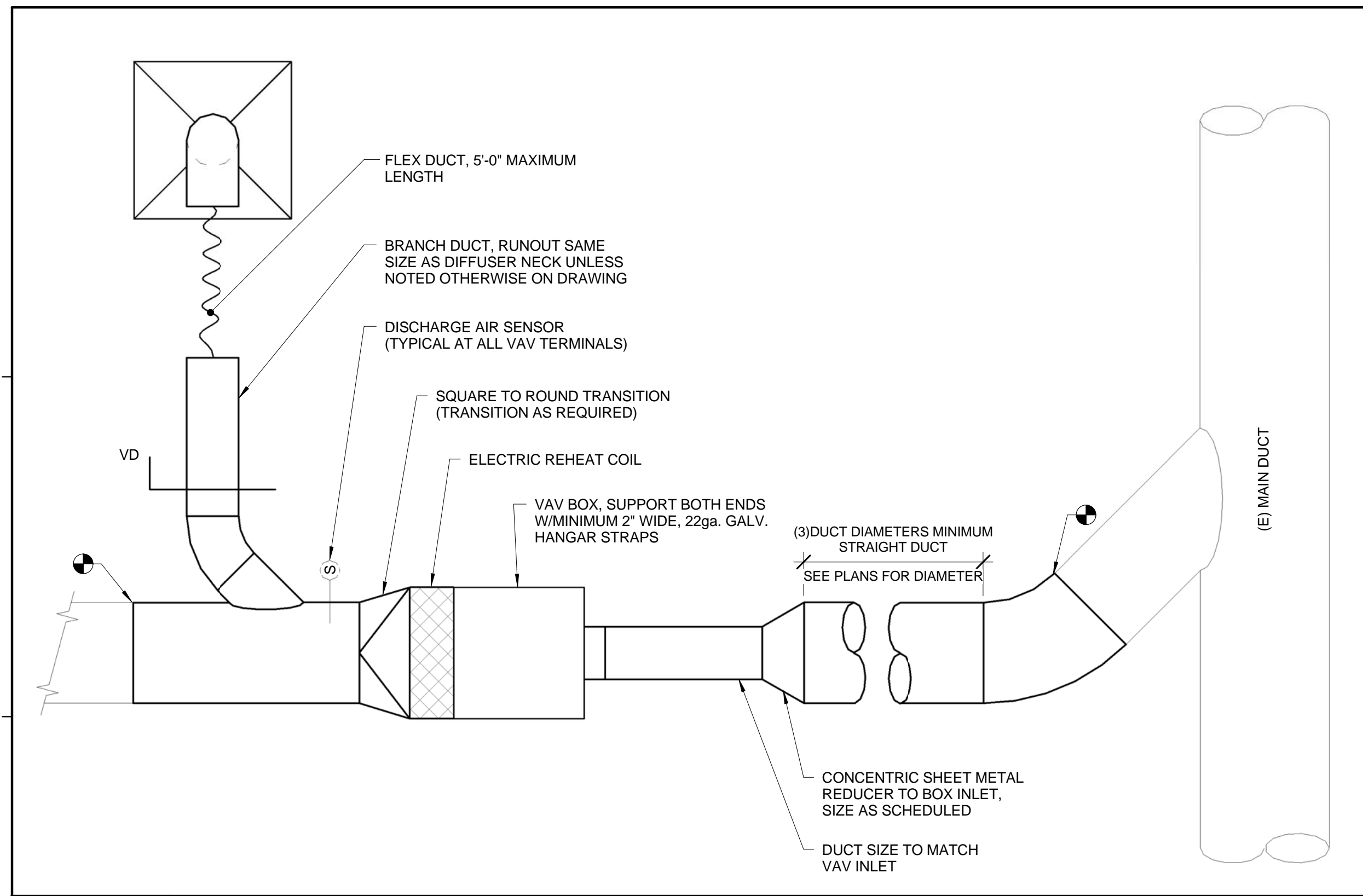
E1 DETAIL - VAV BOX SCHEMATIC
