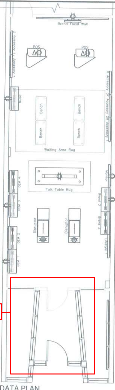
C POWER & DATA PLAN SCALE: 1/8" = 1'-0"
