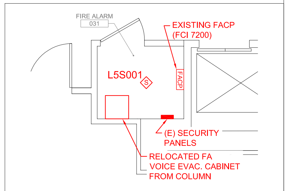
A8 FIRE ALARM ROOM SCALE: 1/4"=1'-0"
