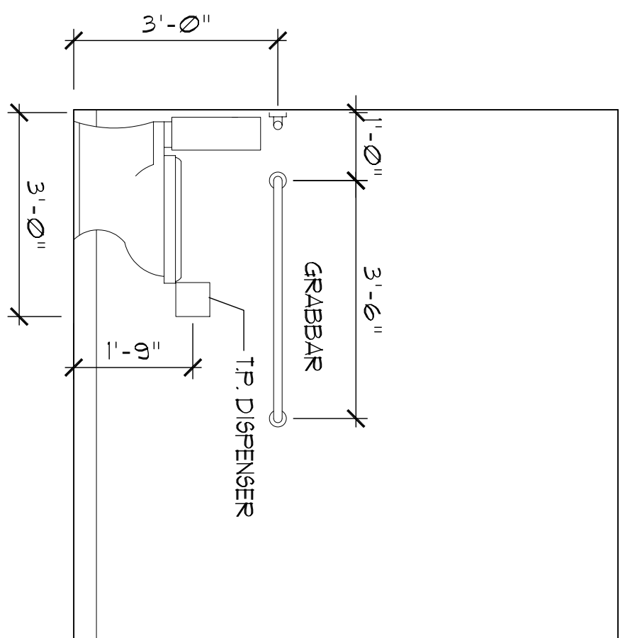
5 BATHROOM ELEV. SCALE: 1/2" = 1'-0"
