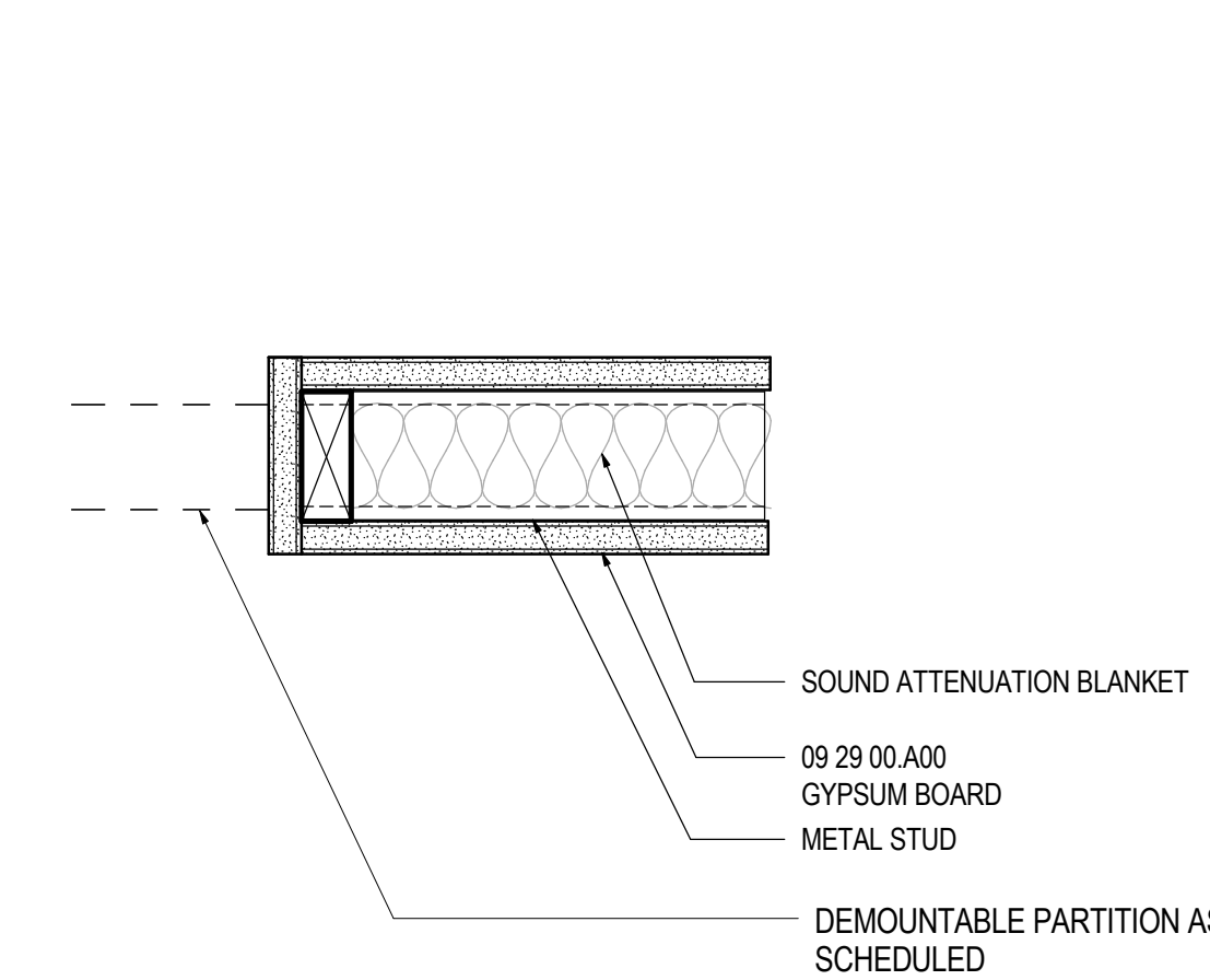
PARTITION JAMB DETAIL Q1
