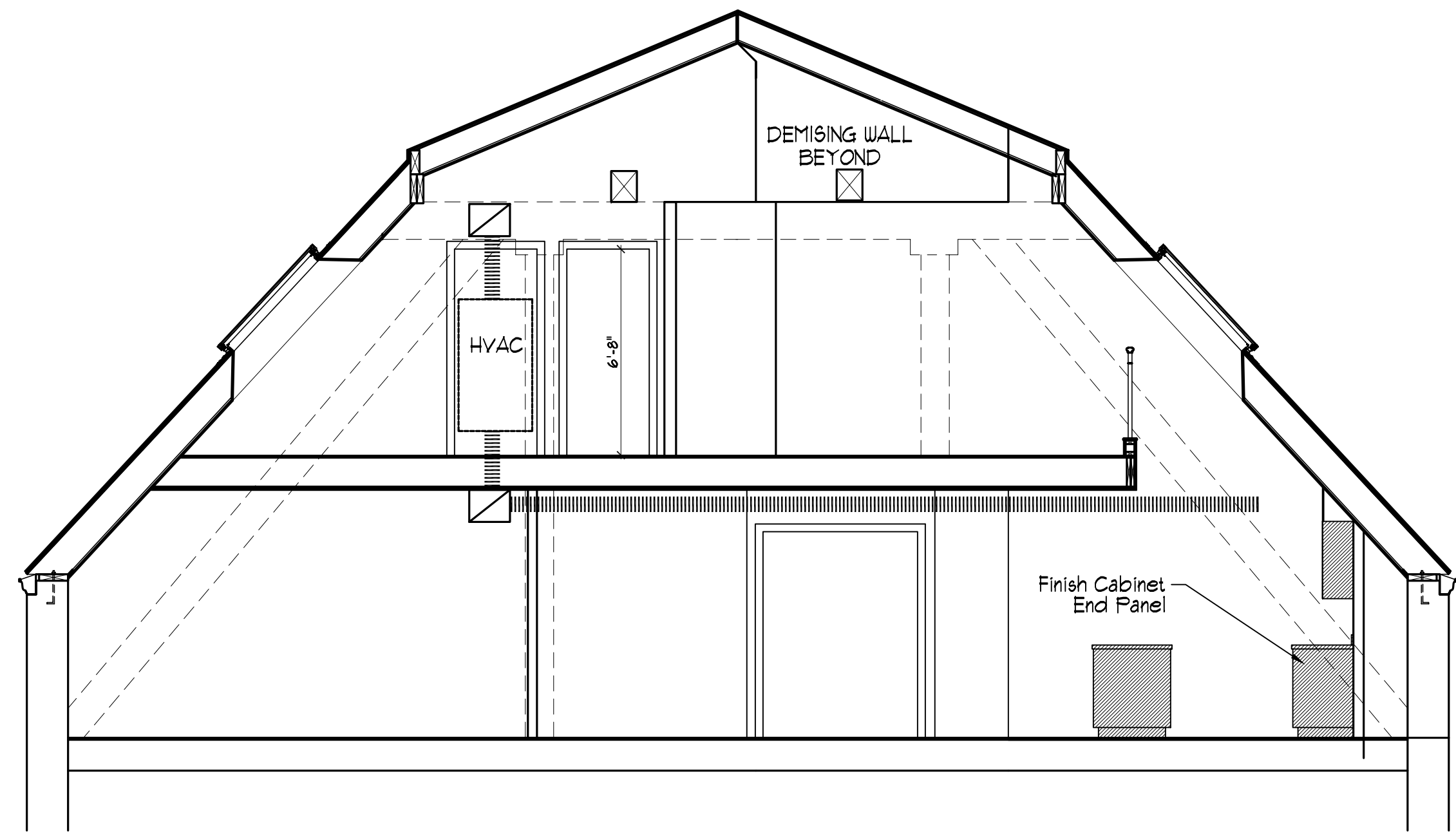
SECTION - UNIT 1 SCALE: 1/4" = 1'-0"
