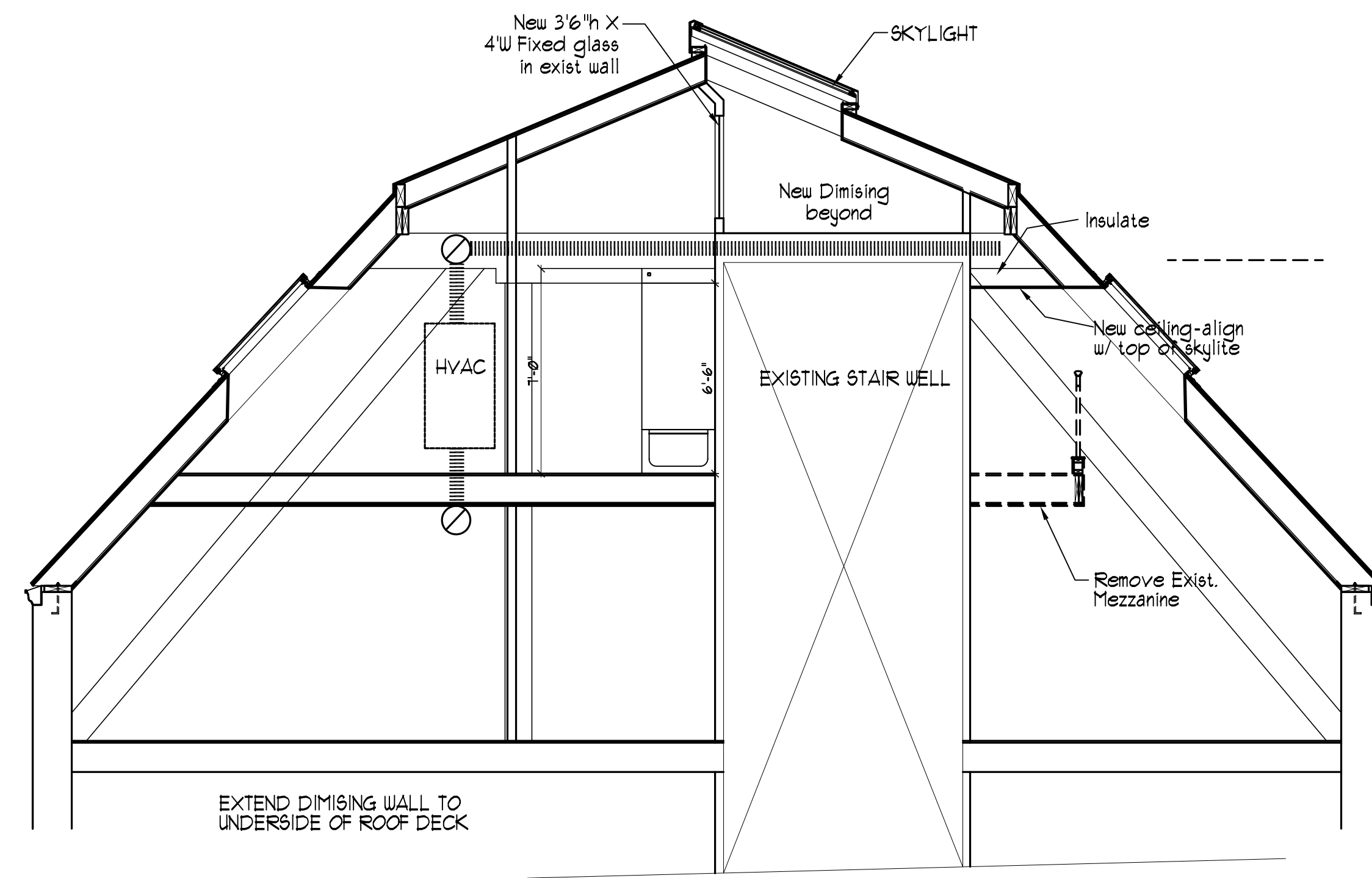
SECTION - UNIT 1 SCALE: 1/4" = 1'-0"
