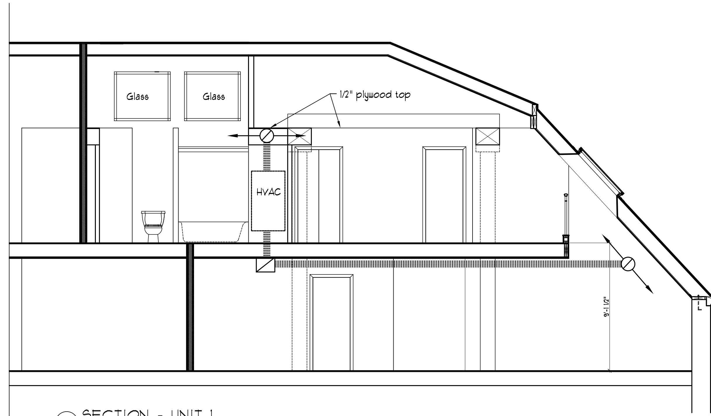
SECTION - UNIT 1 SCALE: 1/4" = 1'-0"
