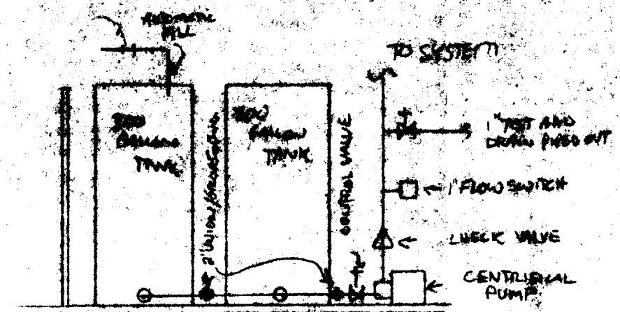
RISER DETAIL N.T.S.
